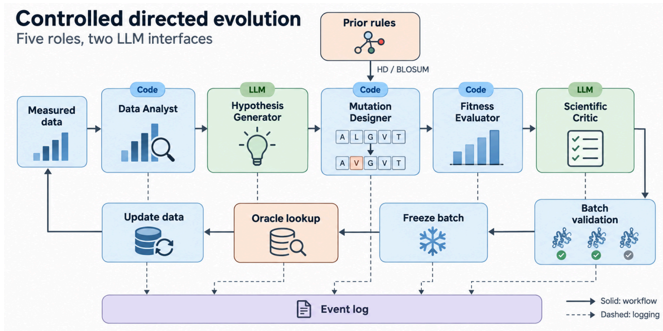
图1 受控定向进化的五角色流程。绿色标签表示两个 LLM 接口, 蓝色标签表示代码模块; 候选批次先校验与冻结, 再查询 Oracle。虚线表示记录流。图表达角色职责与接口边界, 不表示所有历史实验均启用了两个 LLM 接口。
