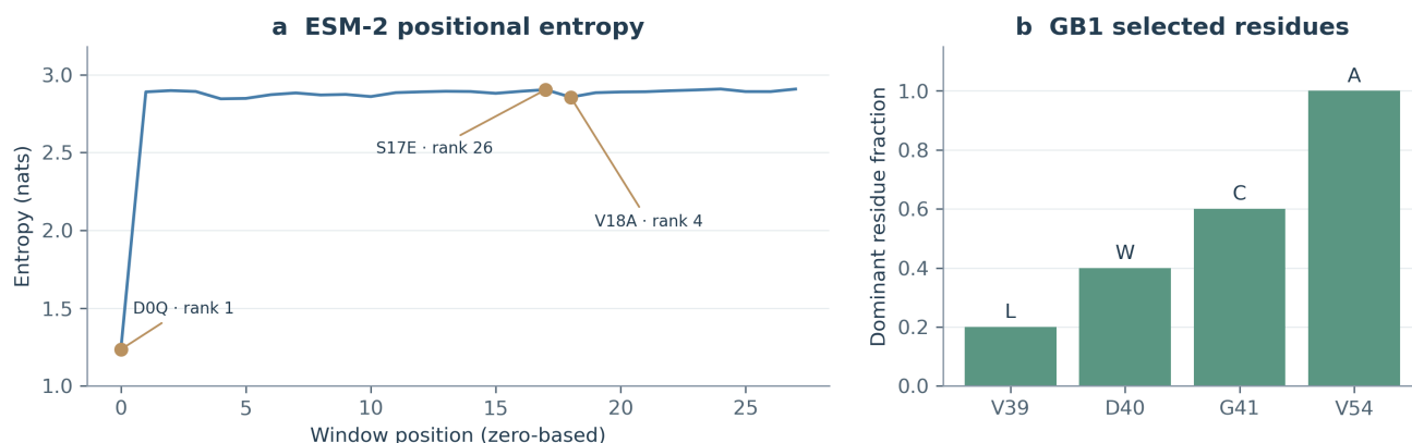
图 7 知识先验与候选组成。左：AAV 位点熵与候选峰的三个替换位置；右：GB1 easy 知识策略三轮 top-10 记录的残基集中度。保守性为事后分析；统计量与坐标约定见附录 G。
