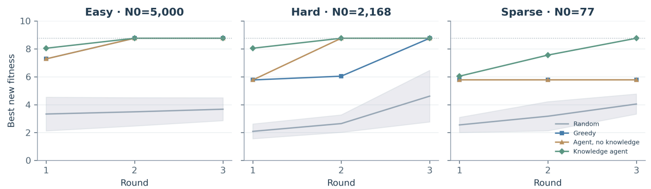
图 4 GB1 不同冷启动的新增最佳适应度。随机曲线为五 seed 均值±总体标准差，其余策略为 seed 42；虚线为全局最优 8.761966。完整预算及语言调用对照见附录 D。
