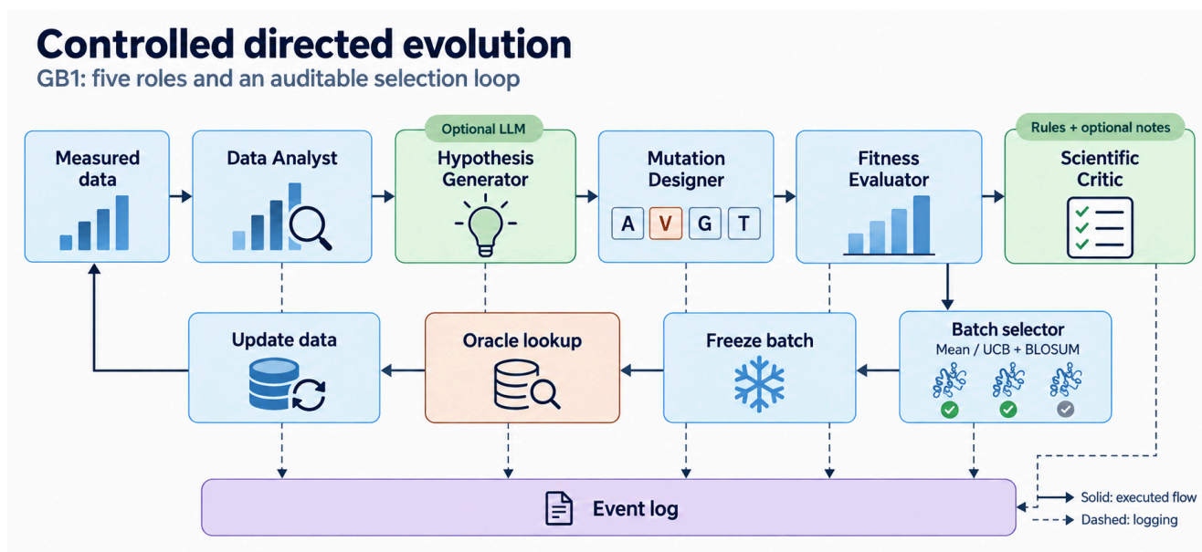
图1 GB1 五角色与实际选样闭环。预测器评分进入批次选择；Critic 判定和评语进入审计记录。角色化执行把假设、候选与测量连接起来。完整接口与消费者接线见附录 C。
