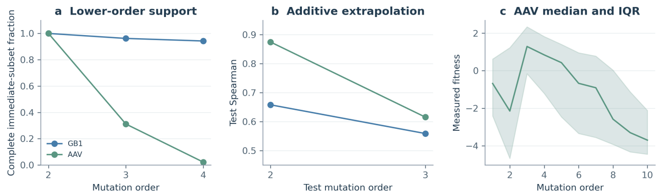
图 S5 突变阶数分析。左：所有直接 (k-1) 阶组成变体均有测量的比例；中：低阶训练向高阶测试的 Spearman；右：AAV 已测样本按 HD 的 fitness 中位数与四分位区间。来源：aav/gb1_mutation_order.json。
