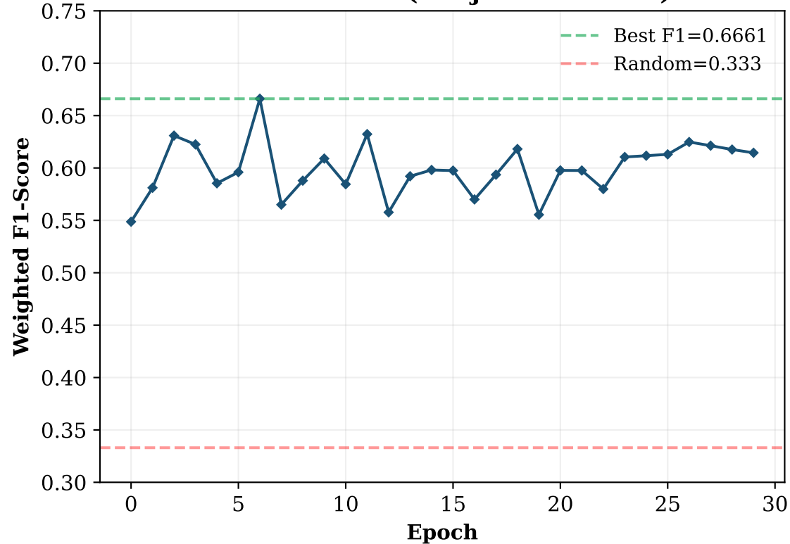
Validation F1 (Subject-Held-Out)
