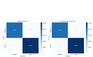
Gambar 3. Confusion Matrix XGBoost (kiri) vs. RF (kanan) pada K=30.
