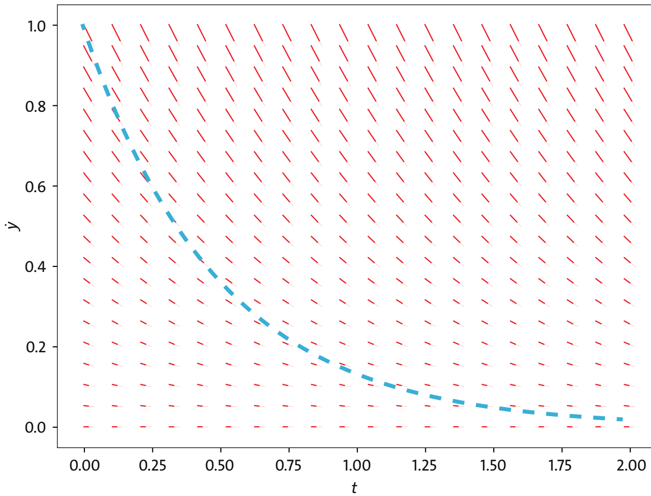
Richtungsfeld
