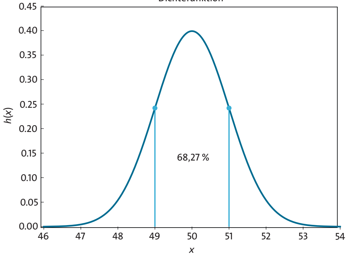
Dichtefunktion
