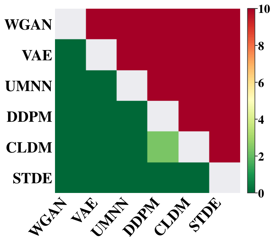
(d) VS DM test.
