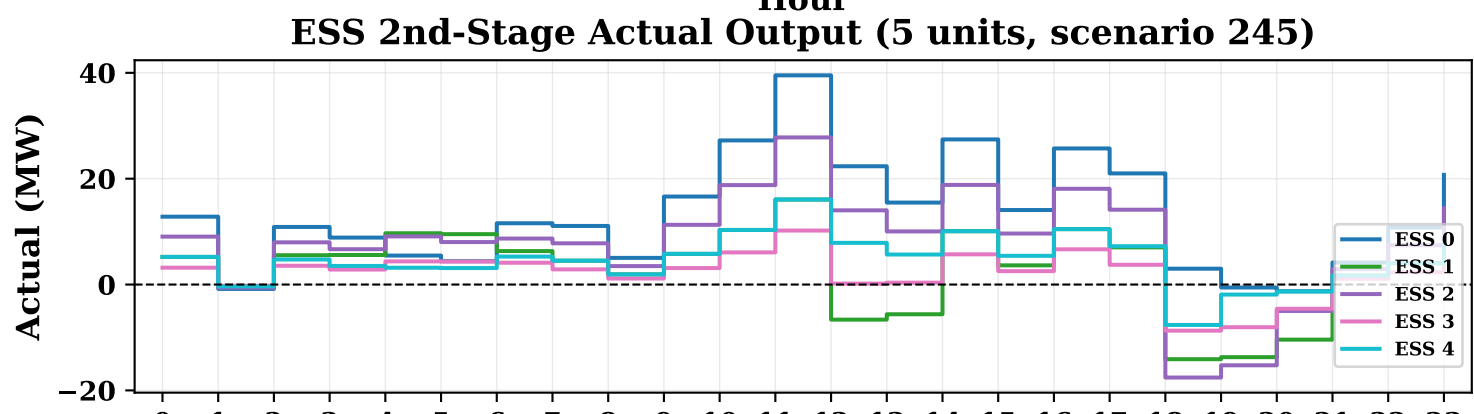
ESS 2nd-Stage Actual Output (5 units, scenario 245)
