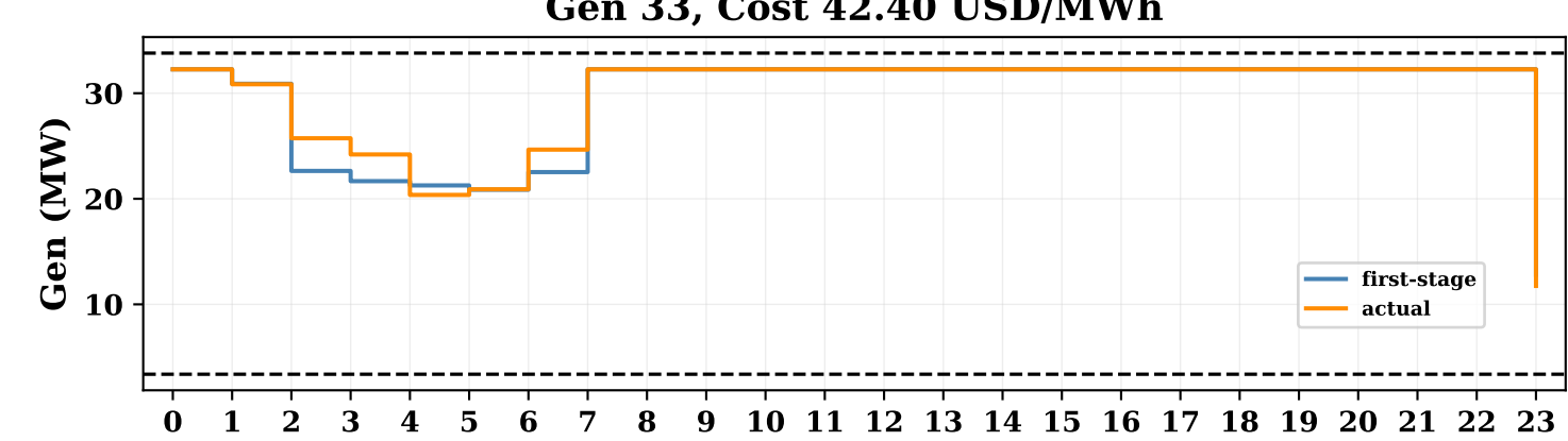
Gen 33, Cost 42.40 USD/MWh
