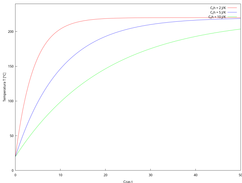
Rysunek 4: Wpływ C_{th} na szybkość nagrzewania
