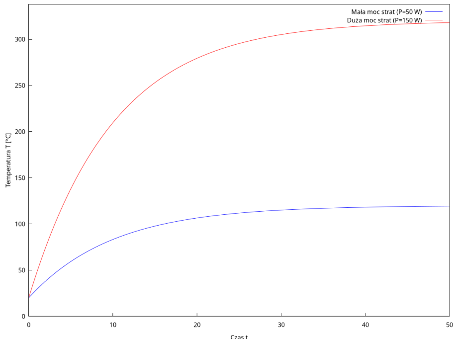
Rysunek 2: Przebieg temperatury silnika T(t) w czasie dla różnych wartości mocy strat P .
