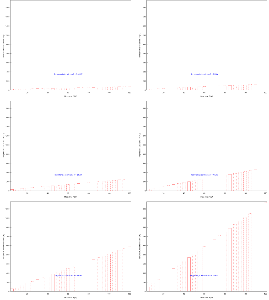
Rysunek 3: Zależność temperatury ustalonej T_{\infty}(P) dla różnych wartości rezystancji termicznej R_{th} .
