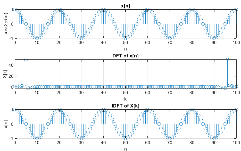
圖(三)、利用 fft 、 ifft 計算結果
