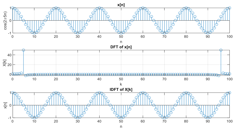
圖(二)、利用 DFT matrix 計算結果
