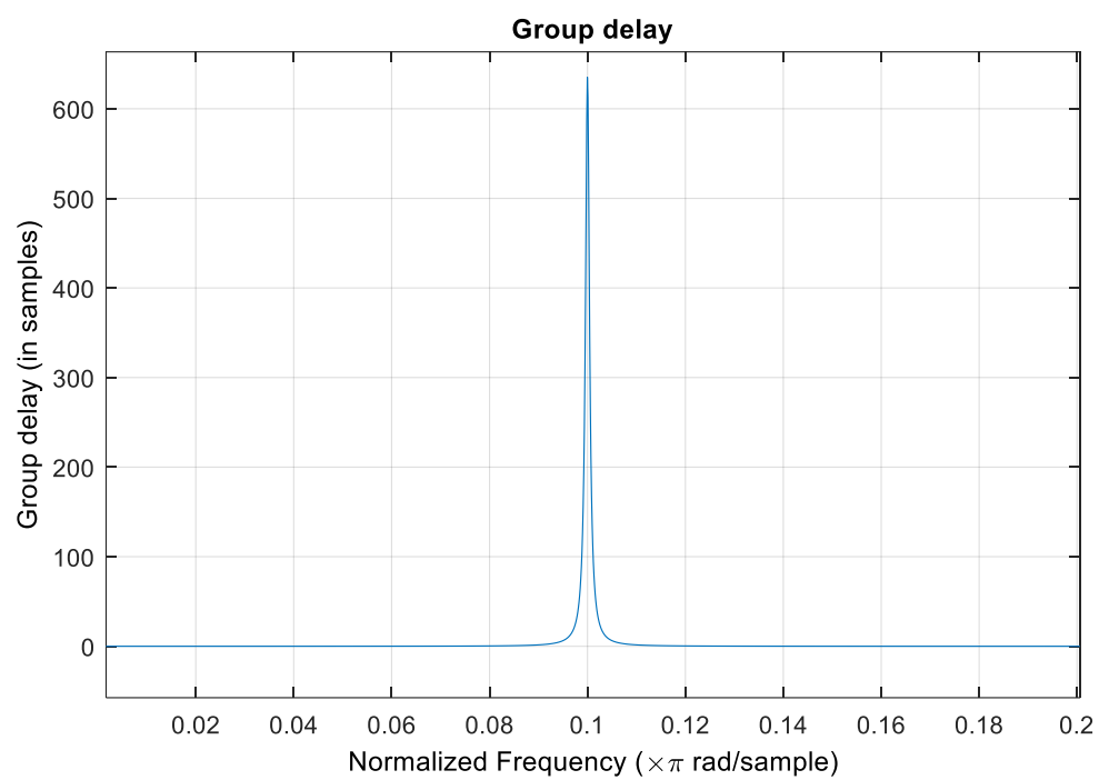
圖(二)、Group delay of IIR notch filter
