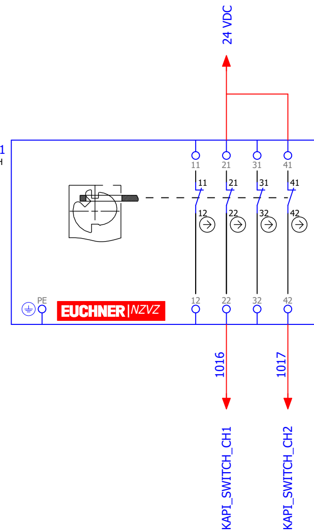
KS1 EUCHNER KAPI SWITCH
