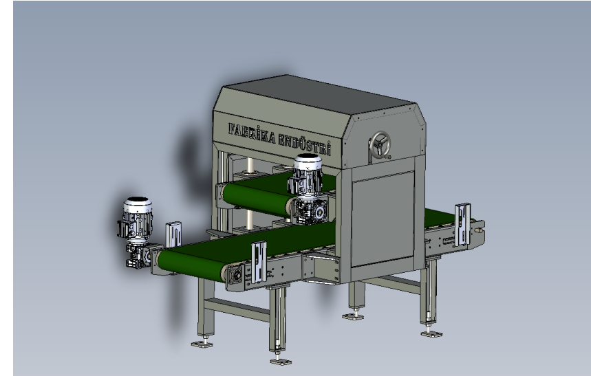
ÜTÜLEME KONVEYÖRÜ
