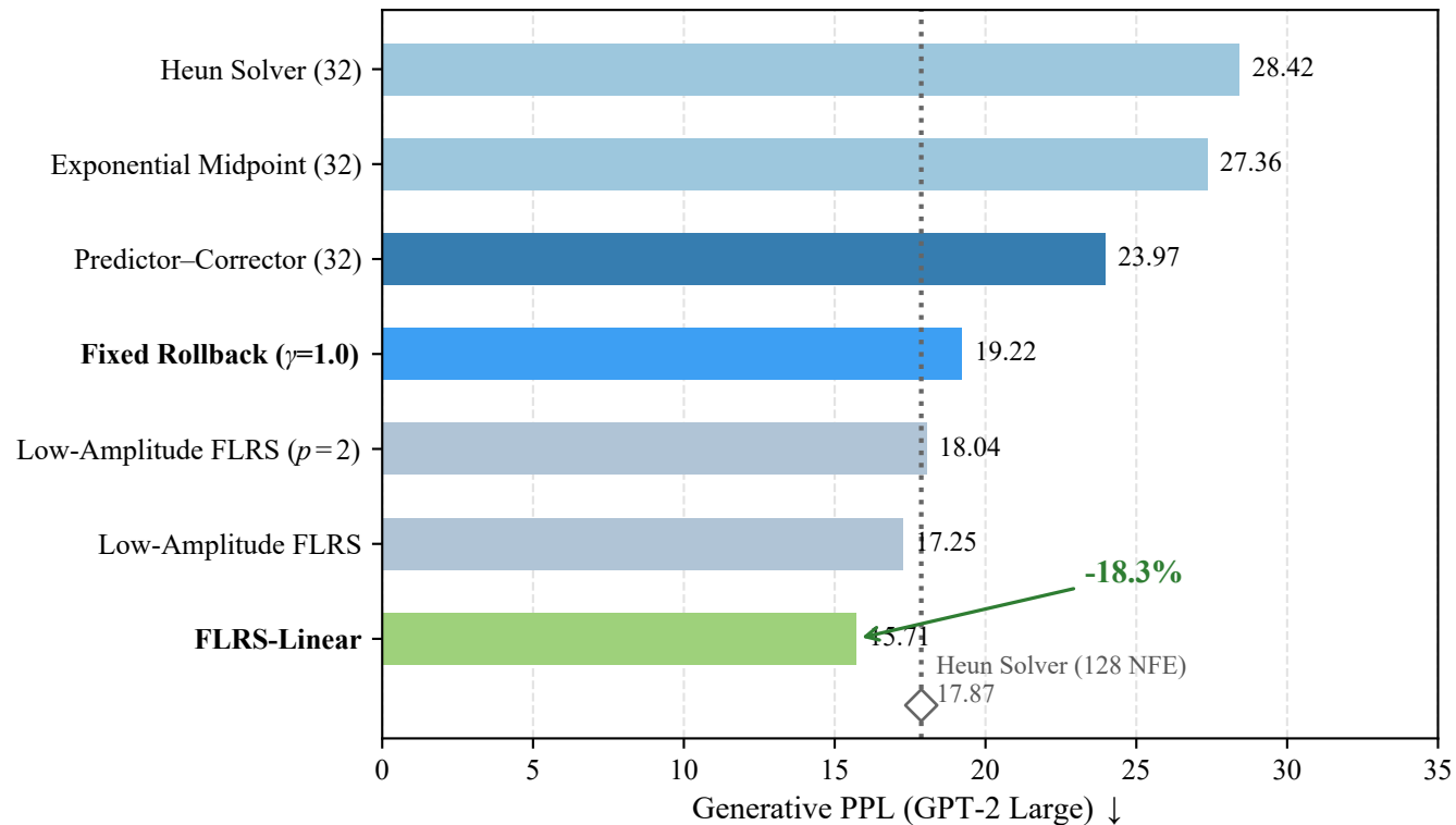
(b) 64-NFE budget
