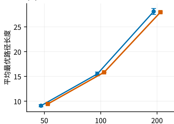
(b) CVRP ↓
