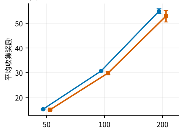
(c) OP ↑
