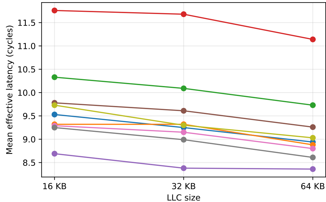
EEMBC
