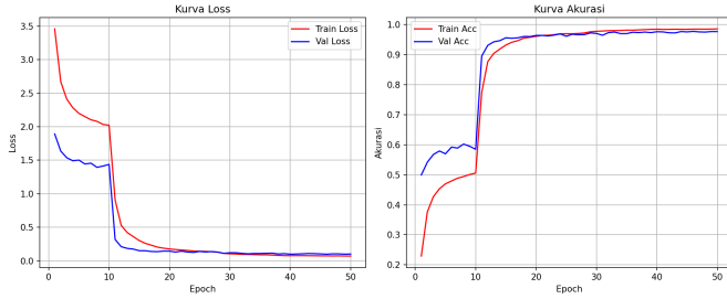
Fig. 2. Kurva pelatihan EfficientNet-B0. Transisi Fase 1 ke Fase 2 terlihat pada epoch 11.
