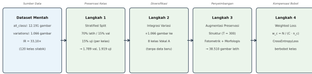
Pipeline Persiapan Data Empat Langkah
