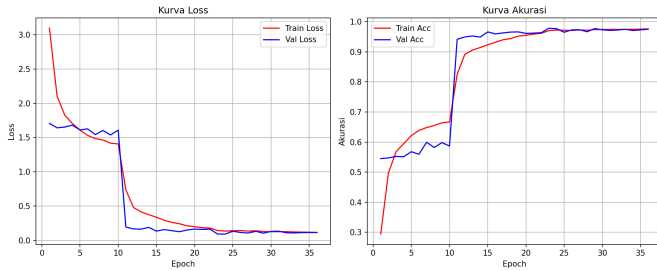
Fig. 3. Kurva pelatihan ResNet-18. Konvergensi yang lebih cepat dibandingkan EfficientNet-B0 (36 vs. 50 epoch).
