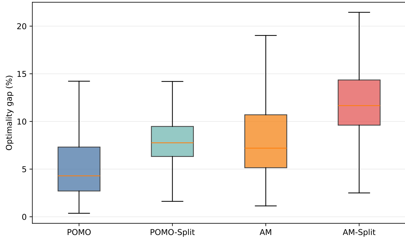
XML100 gap distribution (outliers hidden)
