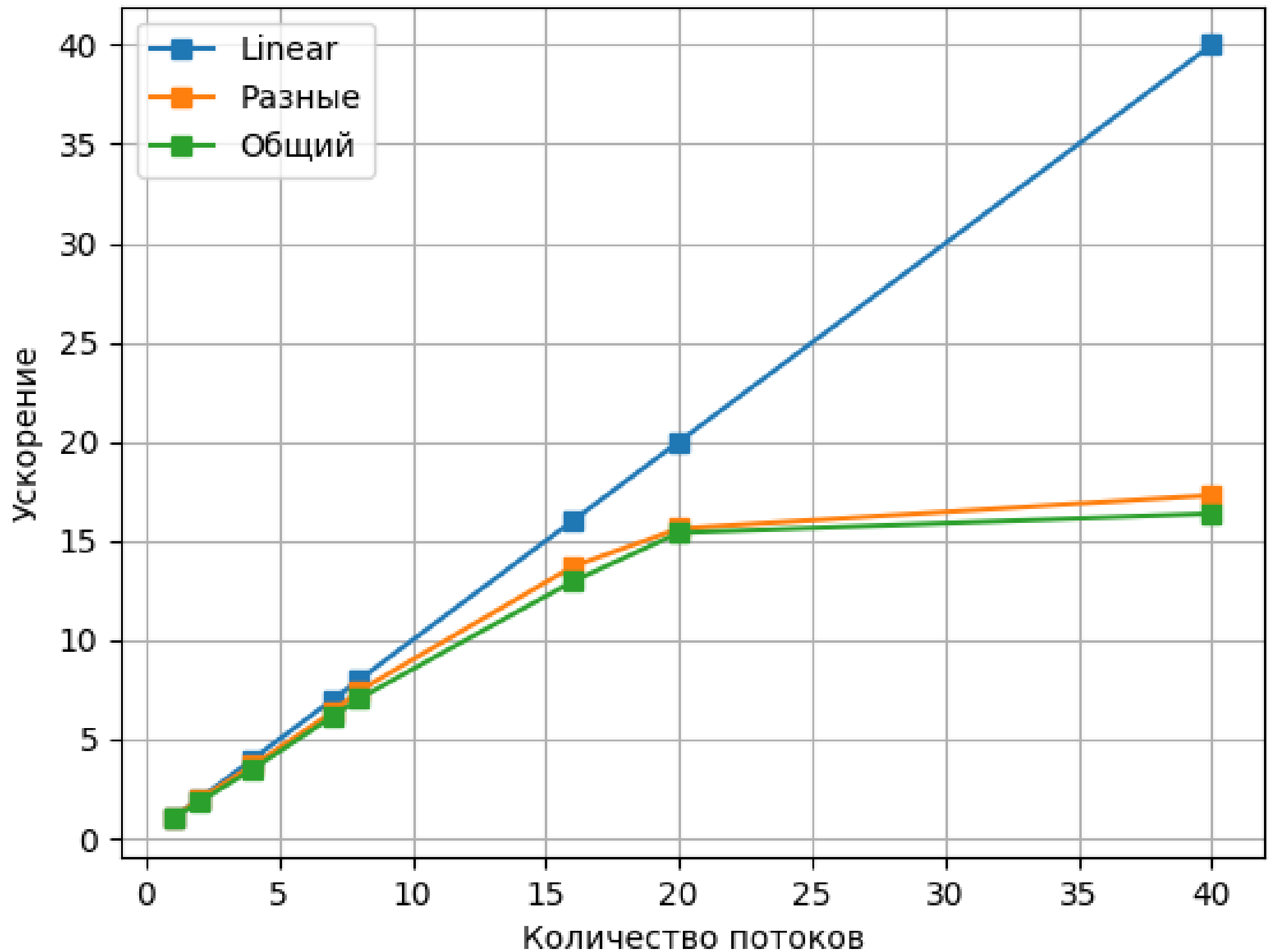
Зависимость ускорения от числа потоков
