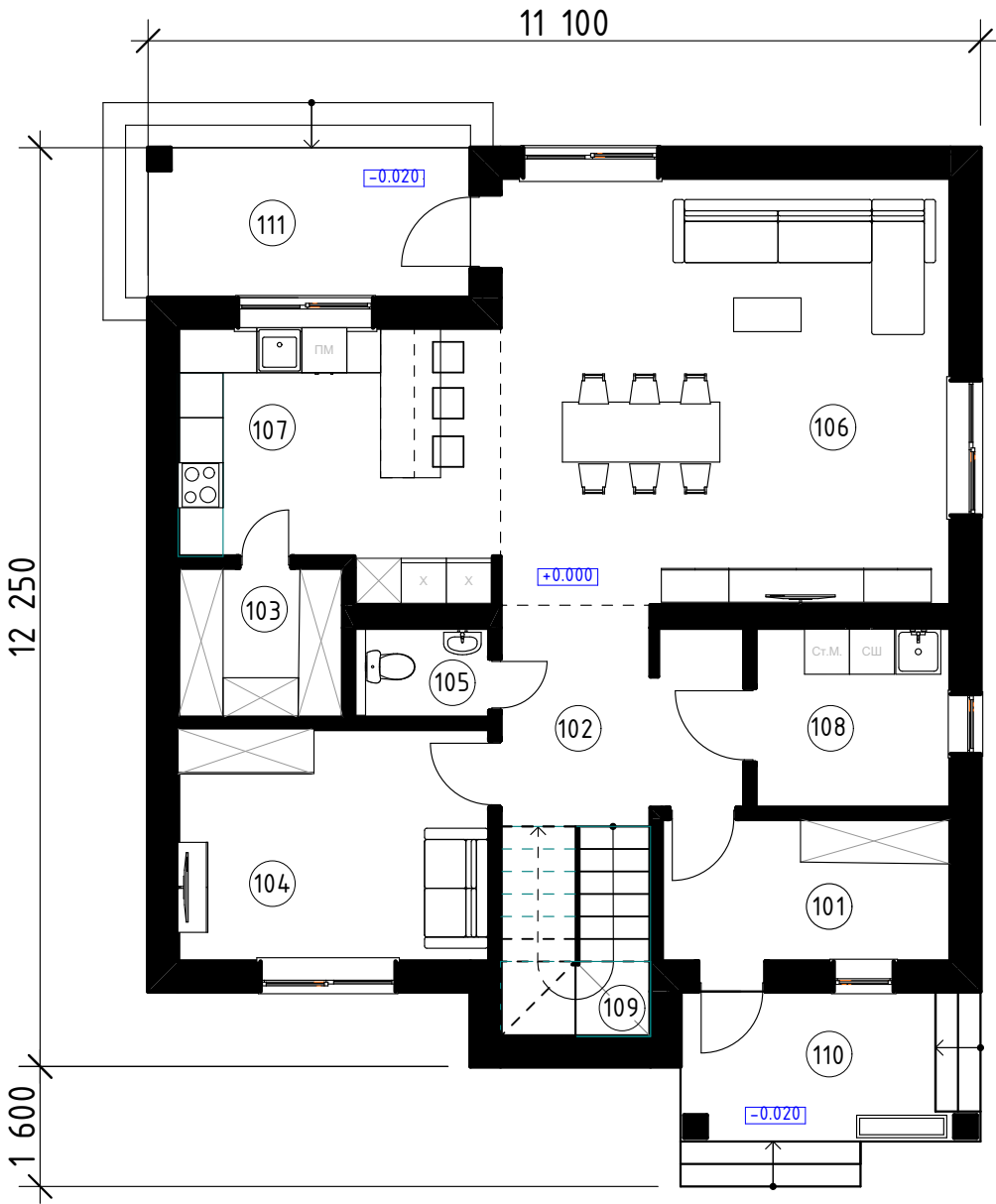
План 1-го этажа
