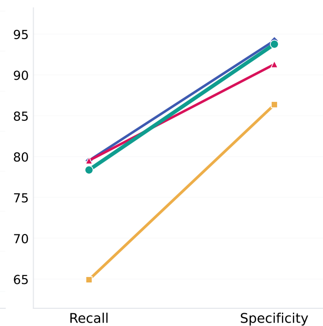
LLaVA-v1.6-Mistral-7B
