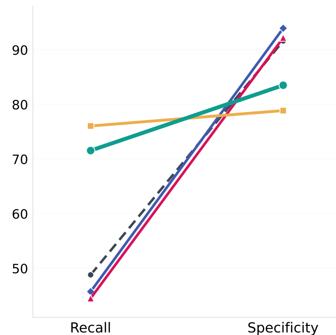
LLaVA-1.5-7B
