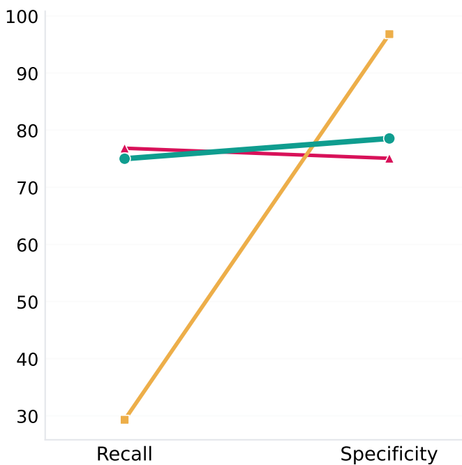
LLaVA-1.5-7B
