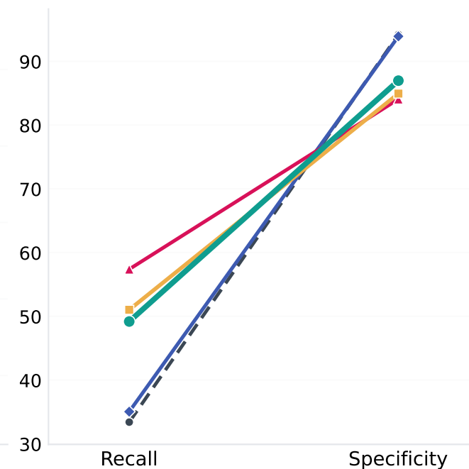
LLaVA-v1.6-Mistral-7B
