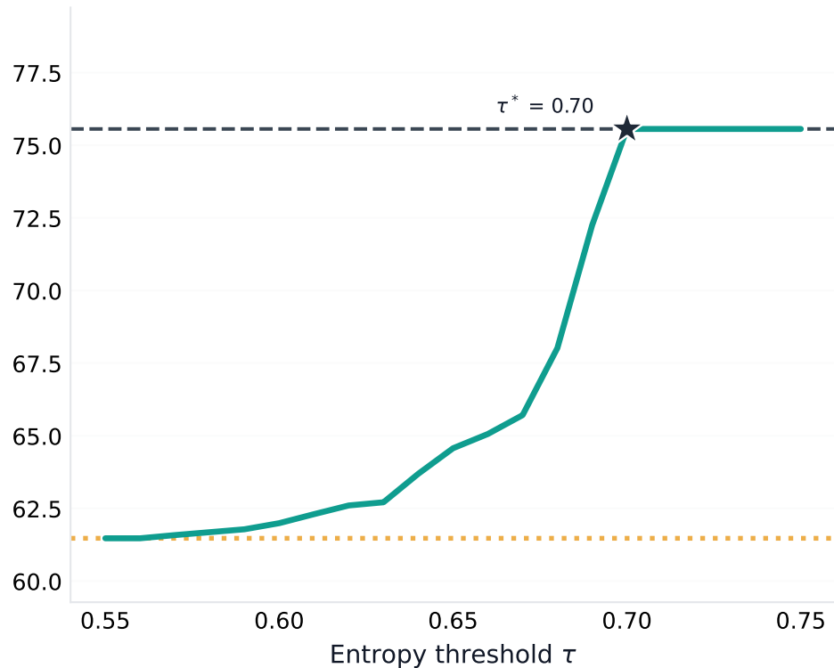
LLaVA-1.5-7B
