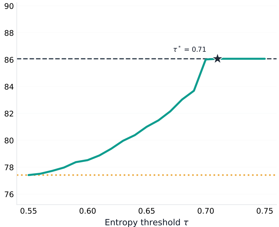
LLaVA-v1.6-Mistral-7B
