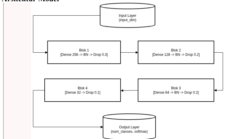
Gambar 4.11 Arsitektur model FCNN
