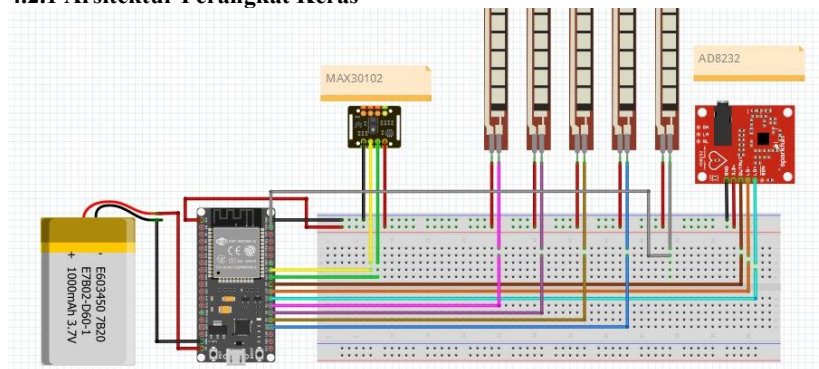
Gambar 4.4 Arsitektur Sistem NeuroRehab Glove AI
