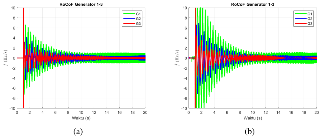
Gambar 4.11. Plot RoCoF dari Gambar 4.10, Gangguan di Bus 1: (a) Skenario 1; (b) Skenario 2
