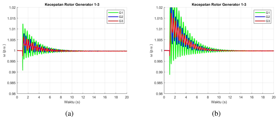
Gambar 4.10. Plot Kecepatan Rotor, Gangguan di Bus 1: (a) Skenario 1; (b) Skenario 2
