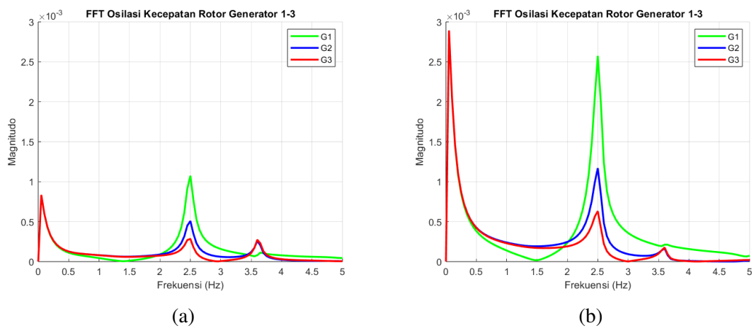
Gambar 4.12. Plot FFT Kecepatan Rotor dari Gambar 4.10, Gangguan di Bus 1: (a) Skenario 1; (b) Skenario 2
