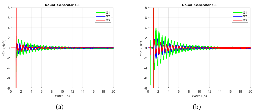
Gambar 4.11. Plot RoCoF, Gangguan di Bus 1: (a) Skenario 1; (b) Skenario 2
