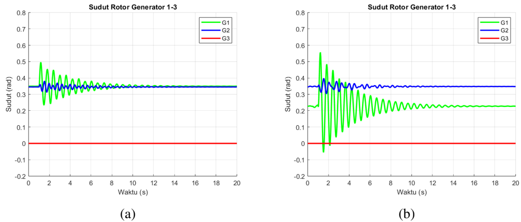
Gambar 4.12. Plot Sudut Rotor, Gangguan di Bus 1: (a) Skenario 1; (b) Skenario 2
