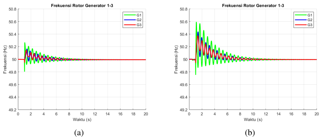
Gambar 4.10. Plot Frekuensi, Gangguan di Bus 1: (a) Skenario 1; (b) Skenario 2
