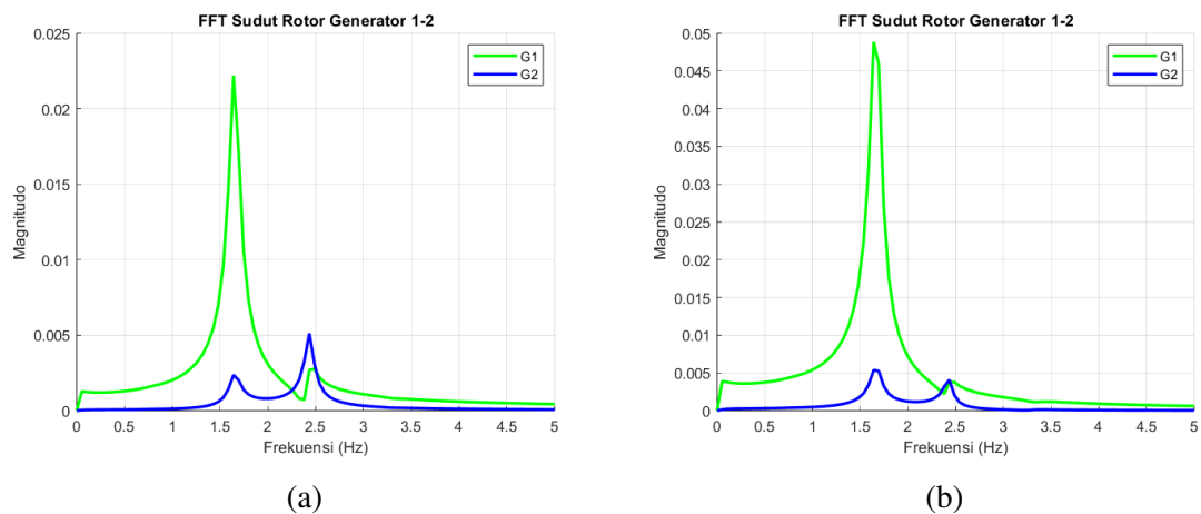
Gambar 4.13. Plot FFT Sudut Rotor, Gangguan di Bus 1: (a) Skenario 1; (b) Skenario 2
