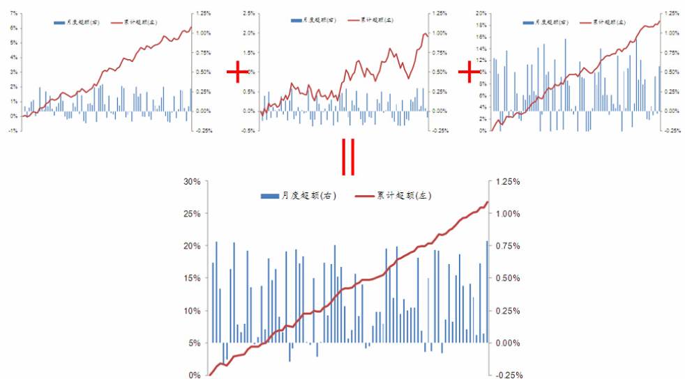
图4 单因子多策略原理
