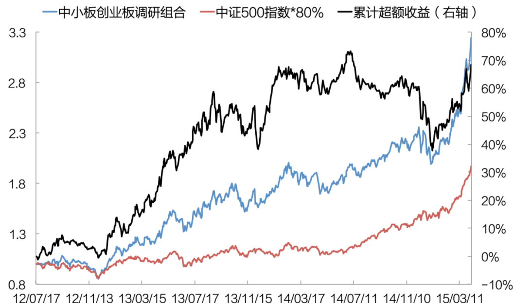
图 2：旧版调研策略使用 80% 中证 500 指数对冲后的表现（截止 2015/04/03）
