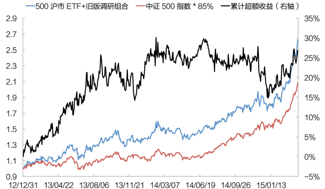
图 7：旧版调研策略对冲后的累计超额收益
