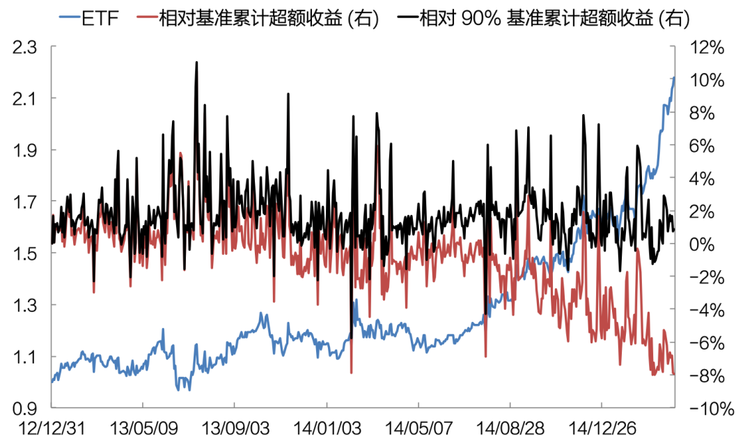
图 5: 中证 500 沪市 ETF 的仓位约为 90%
