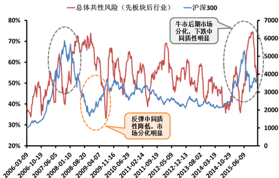
图 17 先板块后行业识别的总体共性风险与指数相关性
