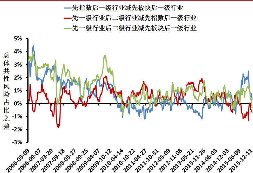
图 16 不同识别因素对市场风险的总体解释度差值
