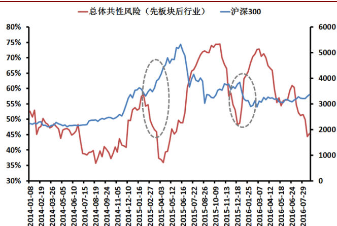
图 18 近期市场总体同质性（截至 2016-8-19）
