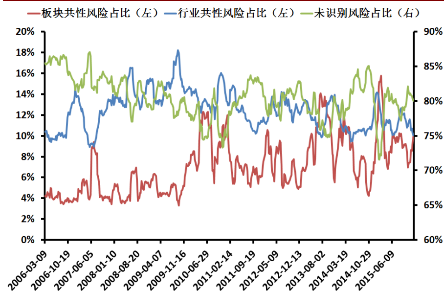
图 10 先板块后行业分层识别的风险占比序列
