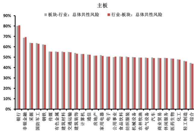
图 5 主板中板块与行业识别次序交换对比
