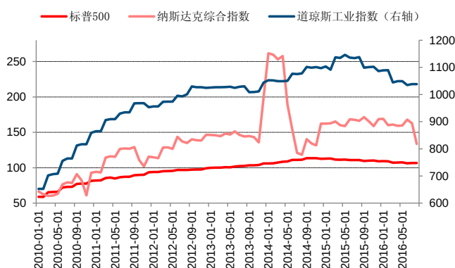
图 1 美股最近 12 个月持续经营所得摊薄每股收益
