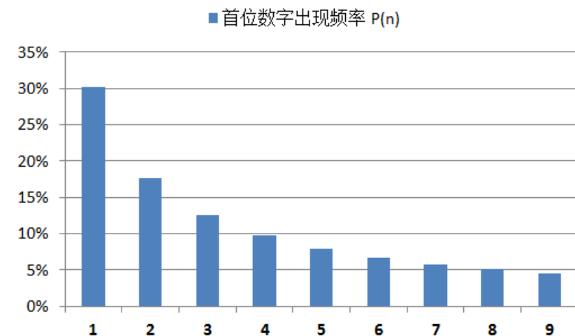
图表 3：本福特法则：首位数字的出现频率
