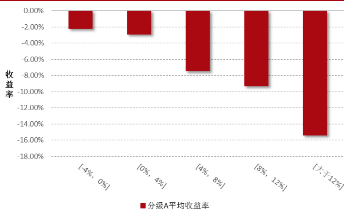
图表 13: 每组分 A 的平均收益率 (T-10 至 T+5)
