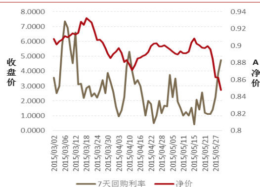
图表 20：分级 A 净价与资金面
