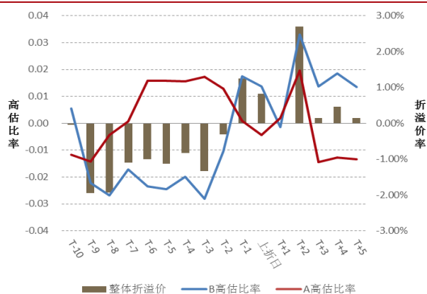
图表 33：信诚中证 800 有色高估比率与整体折溢价率 (2015/04/24 日上折)
