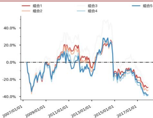
图 20 Leve_cdebt_rat 分层组合走势图（上证 50）
