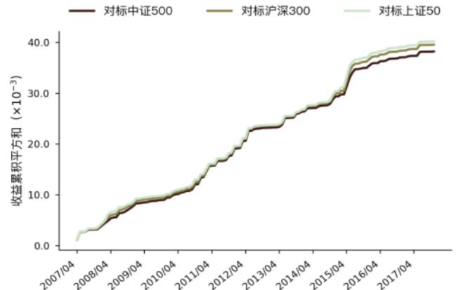
图 29 Leve_cdebt_rat 因子波动量能走势图 (WLS)
