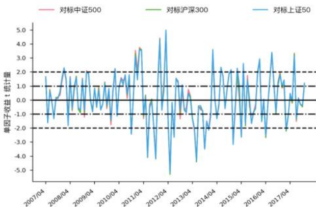
图 28 Leve_cdebt_rat t 统计量走势图 (WLS)
