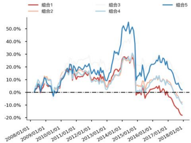
图 115 Liqu_yoy_current 分层组合走势图（沪深 300）
