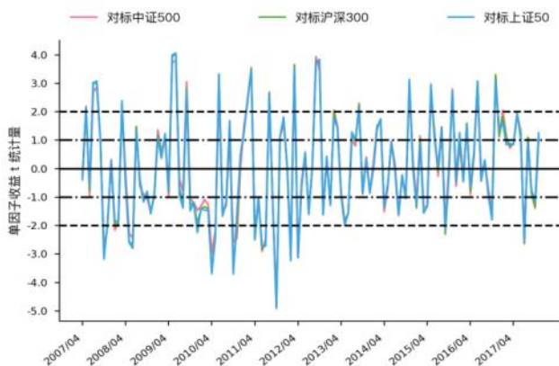
图 88 Liqu_invturn t 统计量走势图 (WLS)
