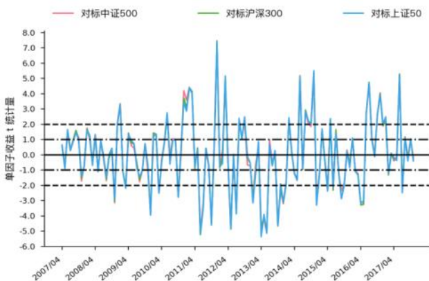
图 16 Leve_as_liab_rat t 统计量走势图 (WLS)
