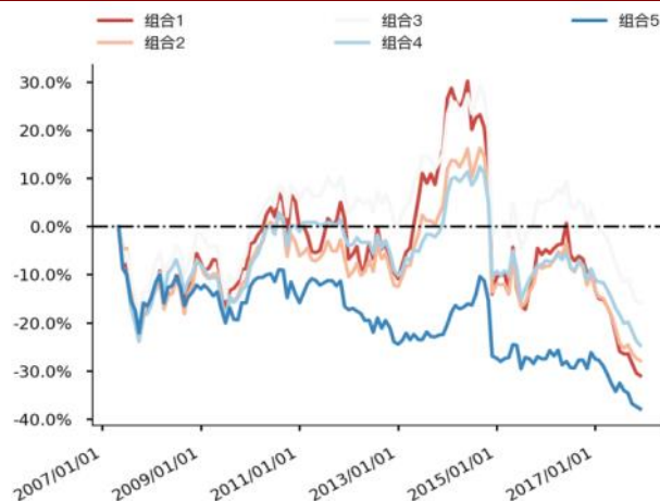
图 67 Liqu_current 分层组合走势图（沪深 300）
