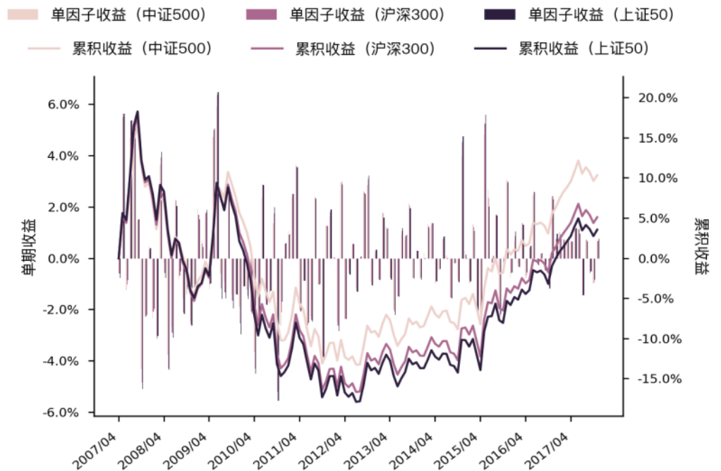
图 87 Liqu_invturn 单因子单期收益与累积收益图 (WLS)
