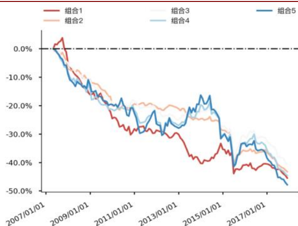
图 6 Leve_as_liab_rat 分层组合走势图（中证 500）
