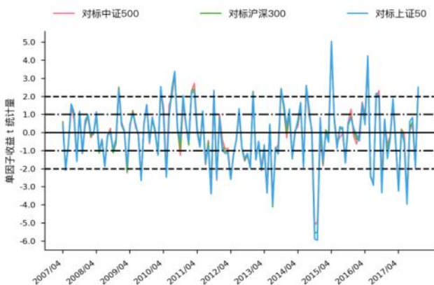
图 40 Leve_fix_rat t 统计量走势图 (WLS)
