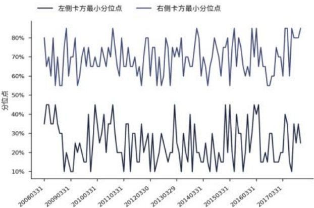
图 142 \chi^2 统计量最小分位点走势（中证 500）
