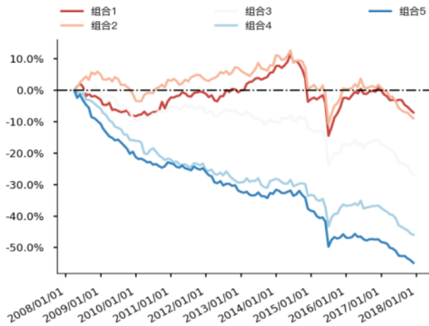
图 126 Liqu_yoy_invturn 分层组合走势图（中证 500）
