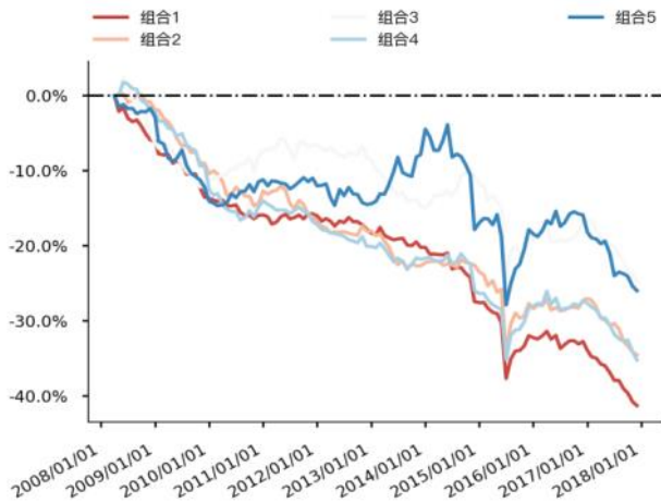
图 114 Liqu_yoy_current 分层组合走势图（中证 500）
