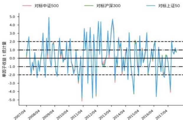
图 76 Liqu_current t 统计量走势图 (WLS)
