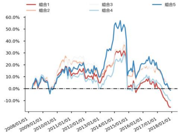
图 139 Liqu_yoy_quick 分层组合走势图（沪深 300）
