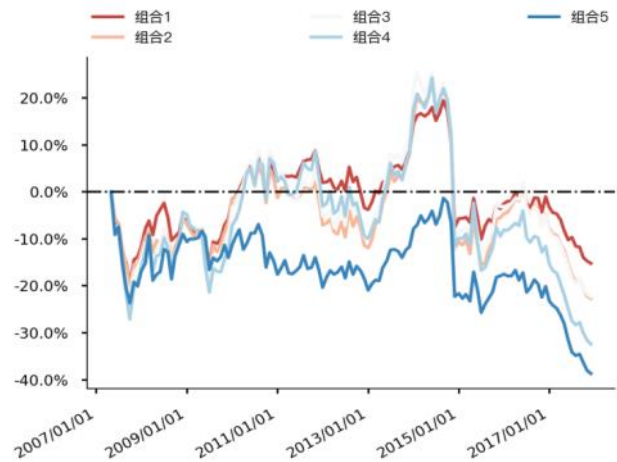
图 79 Liqu_invturn 分层组合走势图（沪深 300）
