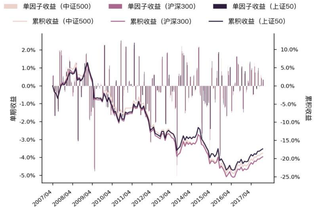
图 51 Leve_ltlebt_rat 单因子单期收益与累积收益图 (WLS)
