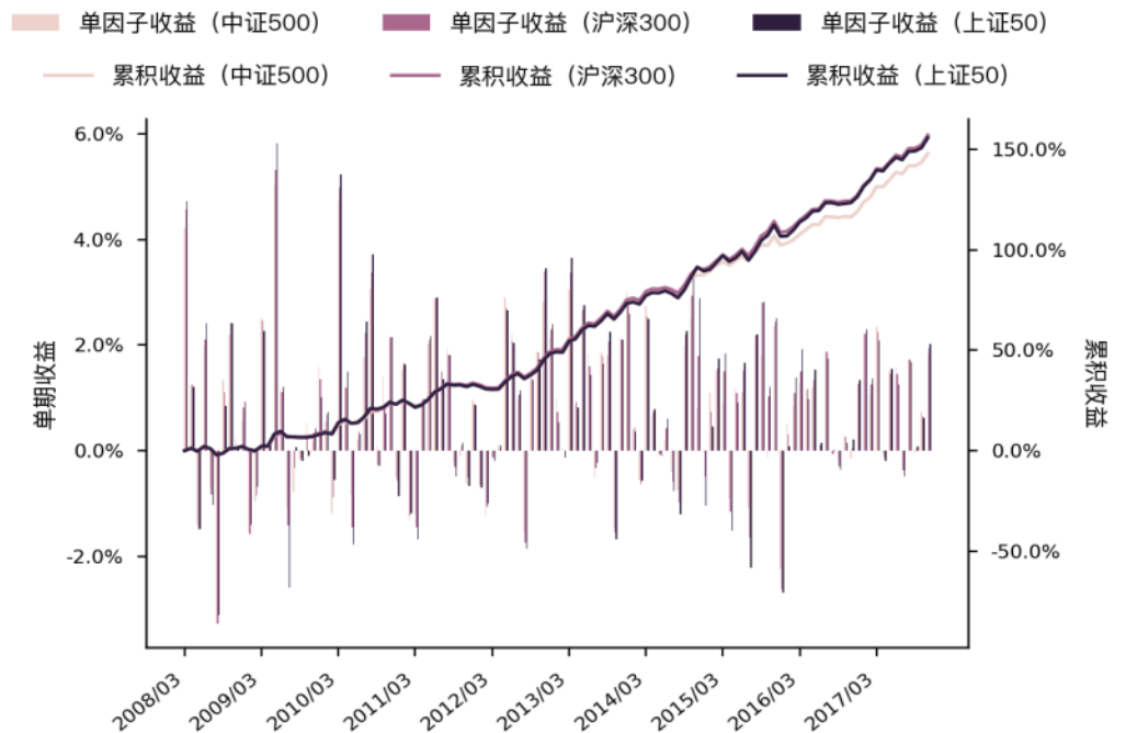
图 111 Liqu_yoy_asturn 单因子单期收益与累积收益图 (WLS)
