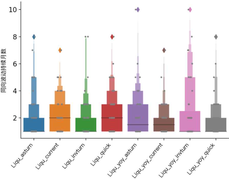
图 153 流动性类因子同向波动持续月份数分布（中证 500）
