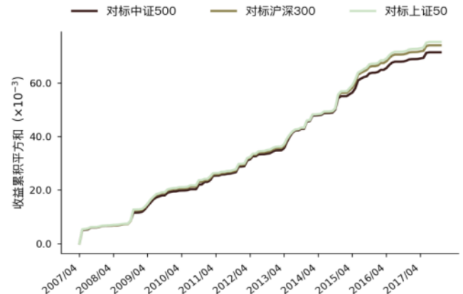
图 101 Liqu_quick 因子波动量能走势图 (WLS)
