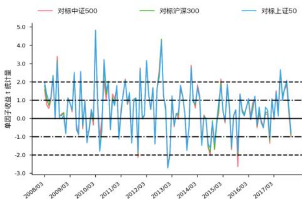
图 136 Liqu_yoy_invturn t 统计量走势图 (WLS)
