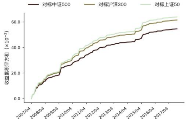
图 89 Liqu_invturn 因子波动量能走势图 (WLS)
