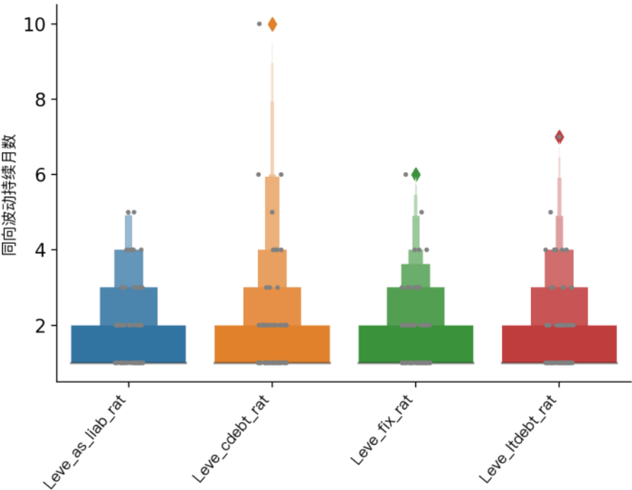
图 151 财务杠杆类因子同向波动持续月份数分布（沪深 300）
