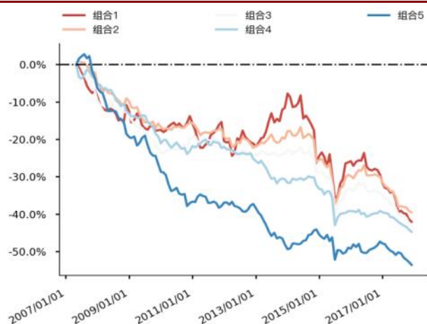
图 90 Liqu_quick 分层组合走势图（中证 500）
