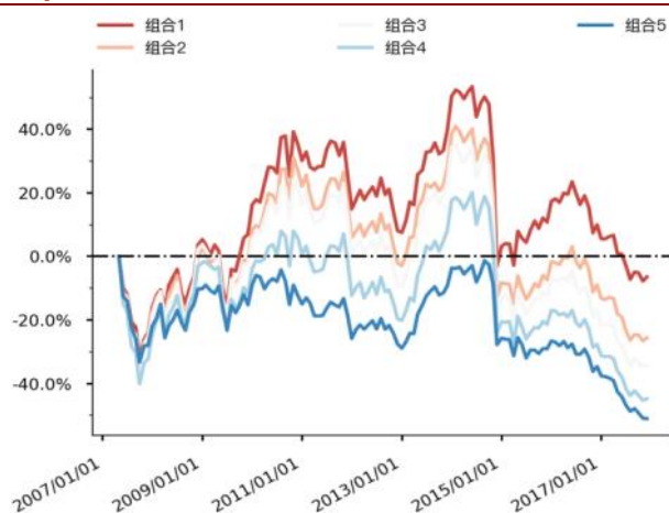
图 56 Liqu_asturn 分层组合走势图（上证 50）
