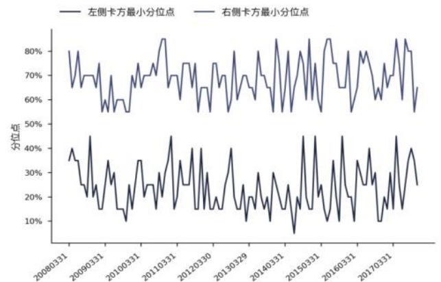
图 121 Liqu_yoy_current \chi^2 统计量分布图 (上证 50) 图 122 \chi^2 统计量最小分位点走势 (上证 50)
