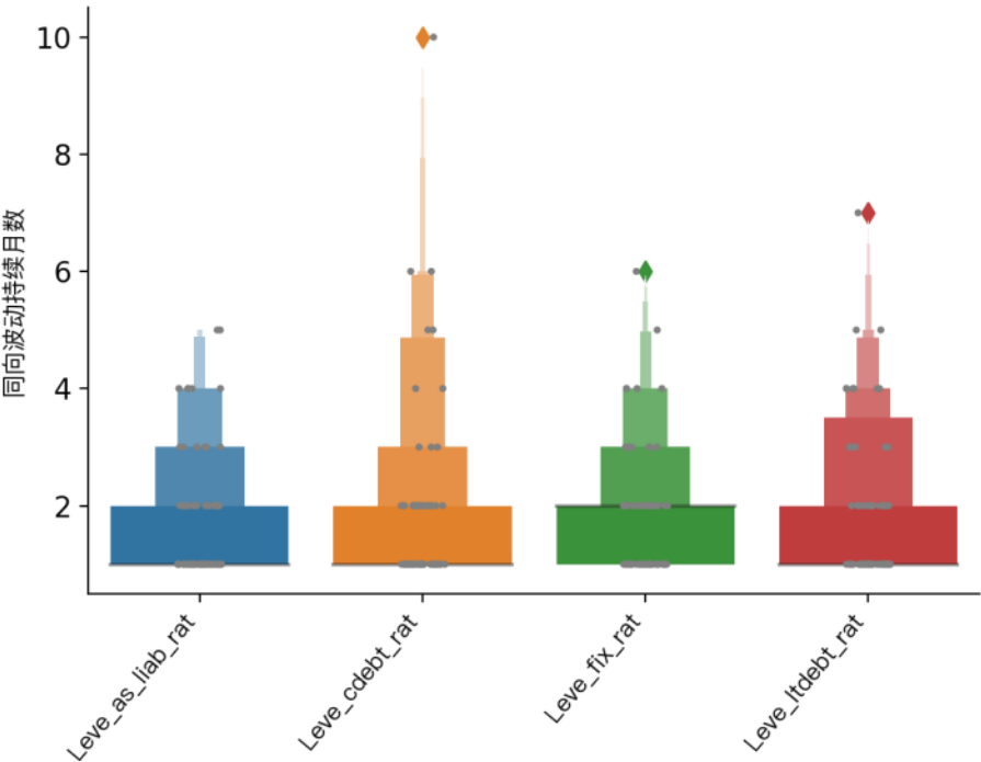
图 152 财务杠杆类因子同向波动持续月份数分布（上证 50）
