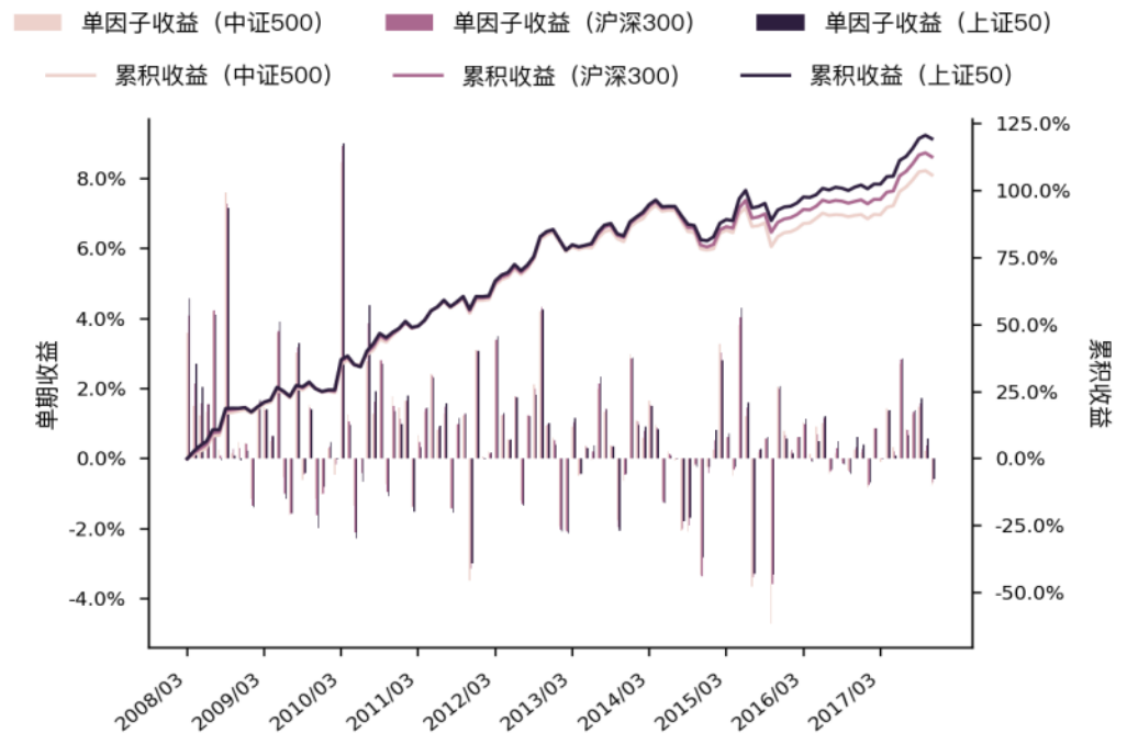
图 135 Liqu_yoy_invturn 单因子单期收益与累积收益图 (WLS)
