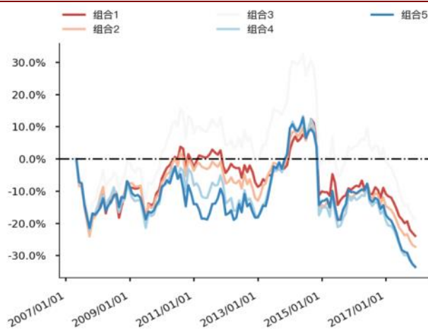
图 19 Leve_cdebt_rat 分层组合走势图（沪深 300）
