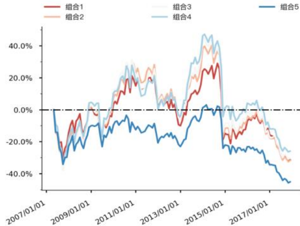
图 32 Leve_fix_rat 分层组合走势图（上证 50）
