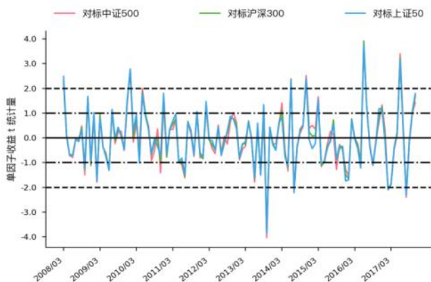
图 124 Liqu_yoy_current t 统计量走势图 (WLS)
