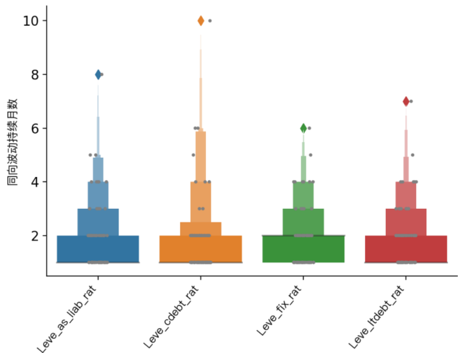
图 150 财务杠杆类因子同向波动持续月份数分布（中证 500）
