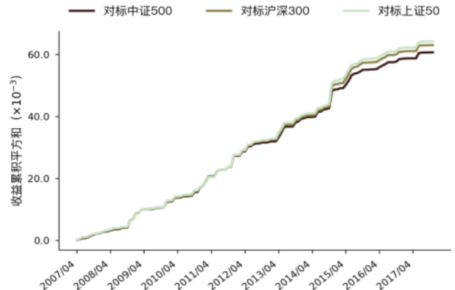
图 17 Leve_as_liab_rat 因子波动量能走势图 (WLS)
