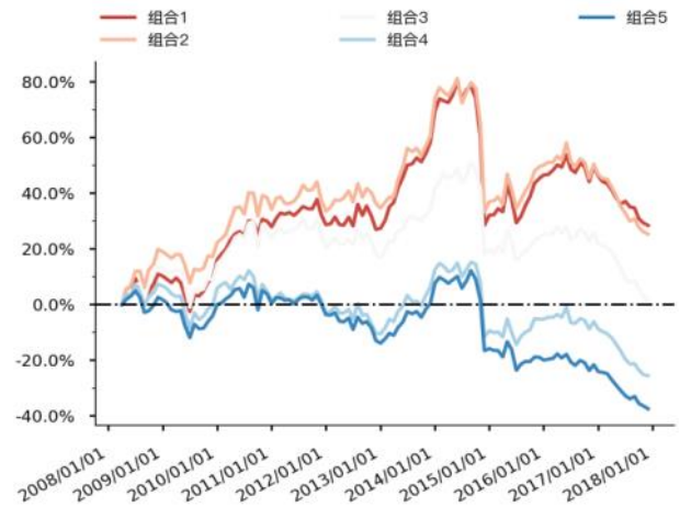
图 127 Liqu_yoy_invturn 分层组合走势图（沪深 300）
