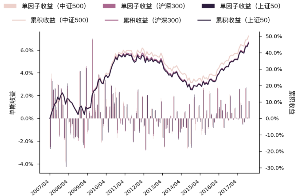
图 63 Liqu_asturn 单因子单期收益与累积收益图 (WLS)
