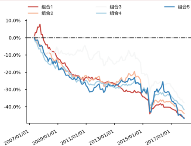
图 42 Leve_ltdebt_rat 分层组合走势图（中证 500）
