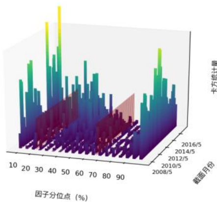
图 143 Liqu_yoy_quick \chi^2 统计量分布图（沪深 300）
