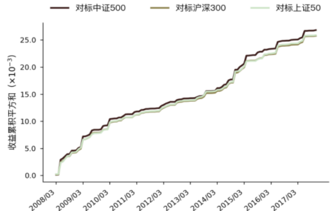
图 149 Liqu_yoy_quick 因子波动量能走势图 (WLS)
