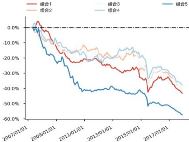
图 30 Leve_fix_rat 分层组合走势图（中证 500）
