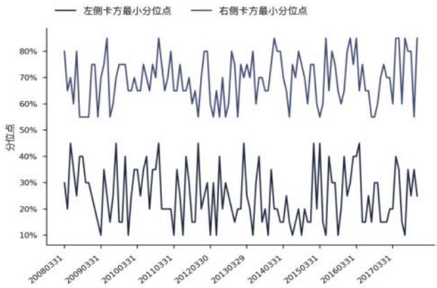
图 146 \chi^2 统计量最小分位点走势（上证 50）
