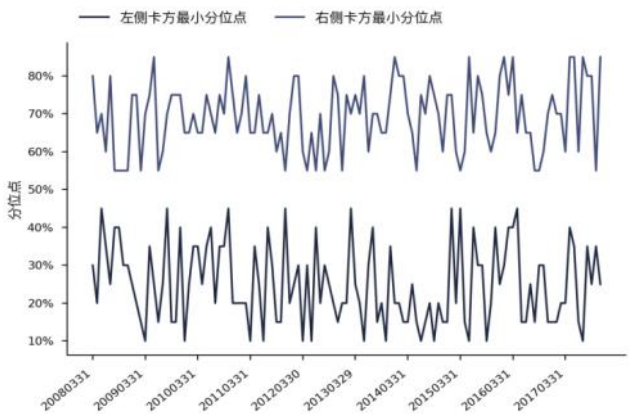
图 144 \chi^2 统计量最小分位点走势（沪深 300）
