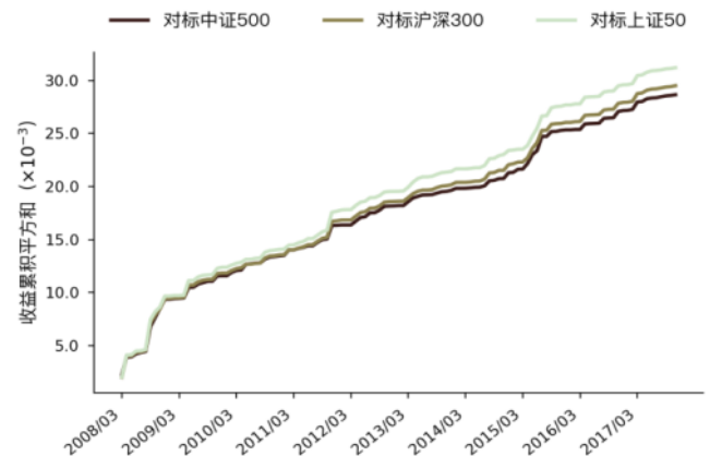
图 53 Grow_asset 因子波动量能走势图 (WLS)
