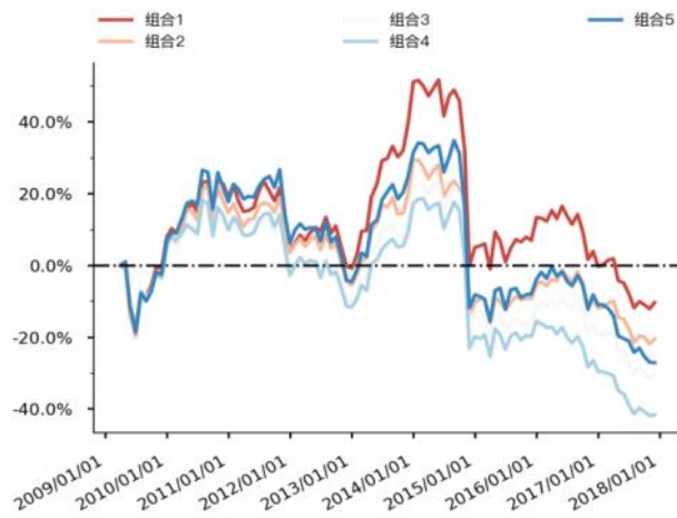
图 116 Grow_yoy_asset 分层组合走势图（上证 50）
