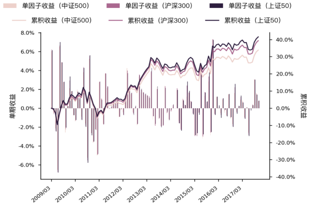
图 111 Grow_yoy_rev 单因子单期收益与累积收益图 (WLS)
