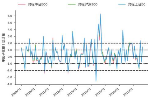
图 136 Grow_yoy_bps t 统计量走势图 (WLS)
