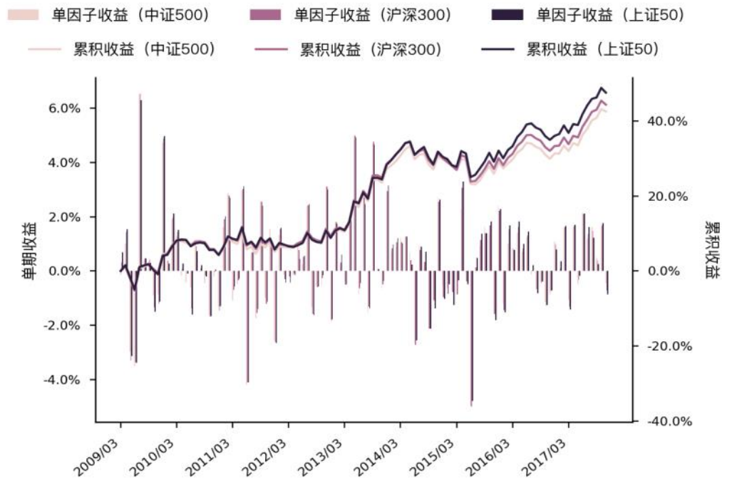
图 87 Grow_yoy_caf_l_op 单因子单期收益与累积收益图 (WLS)
