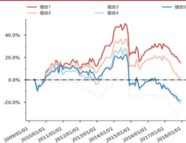
图 127 Grow_yoy_bps 分层组合走势图（沪深 300）
