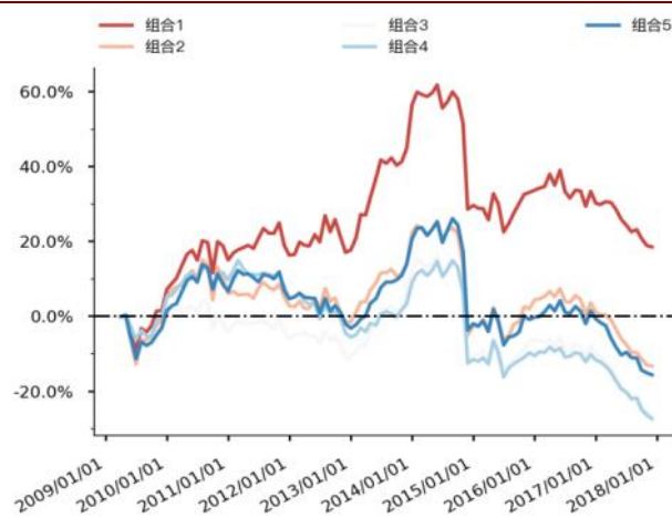
图 103 Grow_yoy_rev 分层组合走势图（沪深 300）
