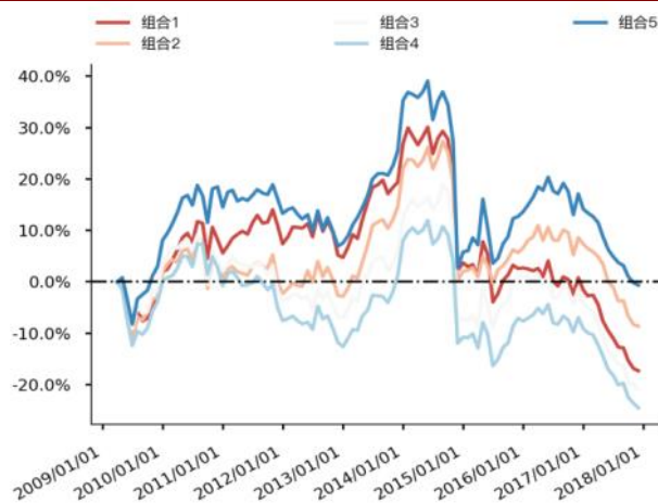
图 139 Grow_yoy_eps_dil 分层组合走势图（沪深 300）
