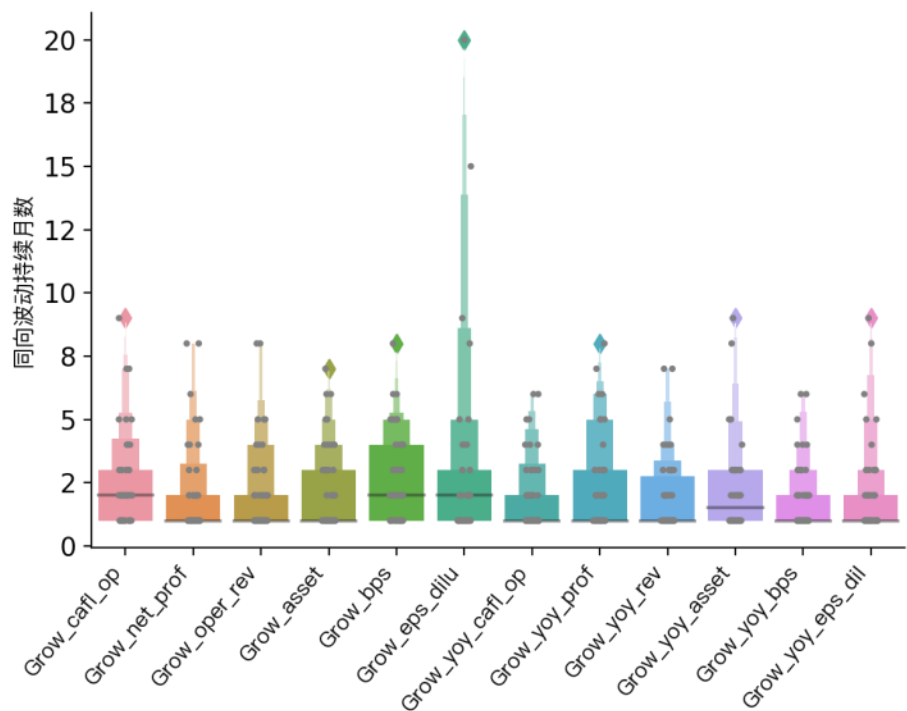
图 152 成长类因子同向波动持续月份数分布（上证 50）
