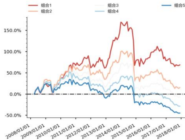
图 32 Grow_oper_rev 分层组合走势图（上证 50）
