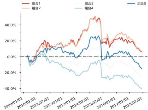
图 91 Grow_yoy_prof 分层组合走势图（沪深 300）
