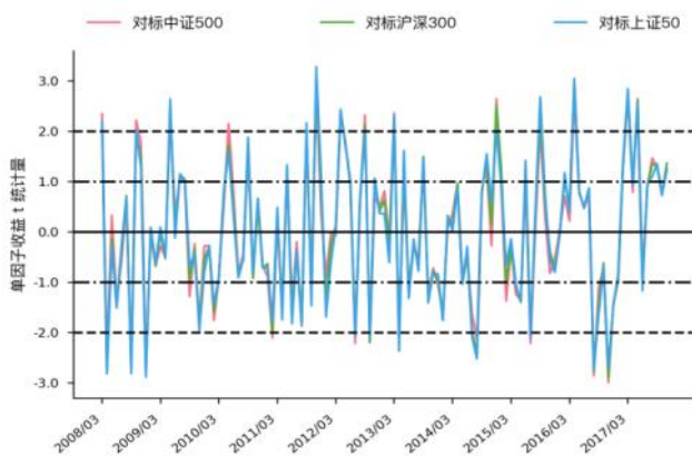
图 52 Grow_asset t 统计量走势图 (WLS)
