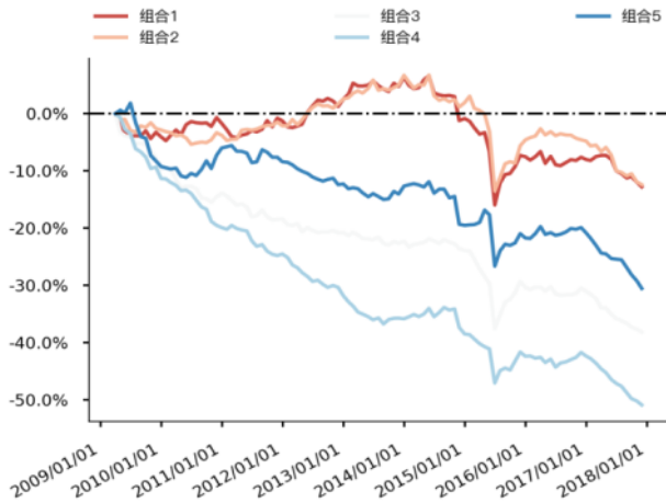
图 90 Grow_yoy_prof 分层组合走势图（中证 500）
