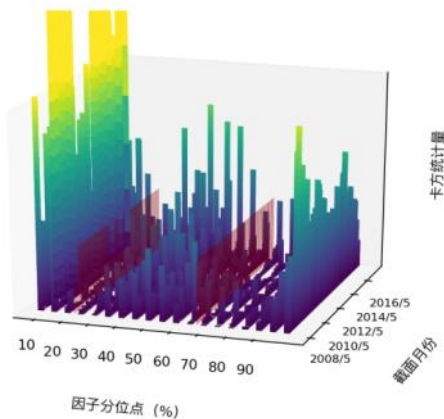
图 45 Grow_asset \chi^2 统计量分布图（中证 500）
