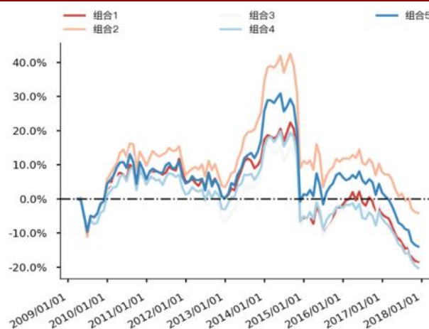
图 79 Grow_yoy_caf_l_op 分层组合走势图（沪深 300）
