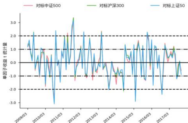
图 148 Grow_yoy_eps_dil t 统计量走势图 (WLS)
