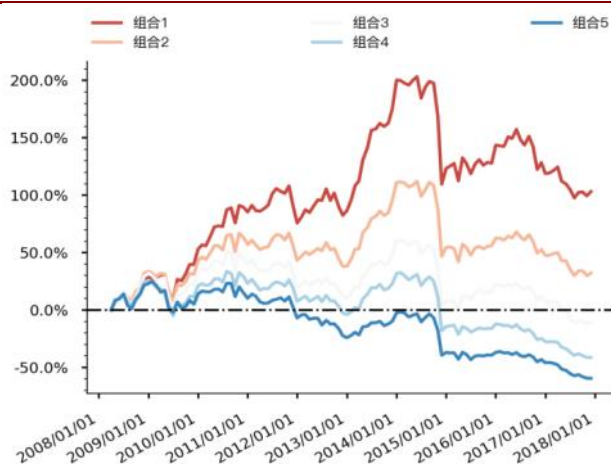
图 68 Grow_eps_dilu 分层组合走势图（上证 50）
