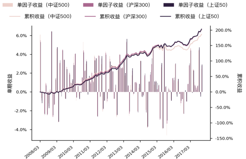
图 27 Grow_net_prof 单因子单期收益与累积收益图 (WLS)
