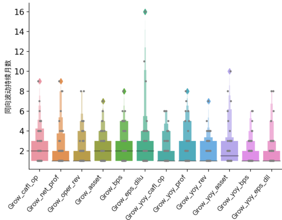
图 151 成长类因子同向波动持续月份数分布（沪深 300）
