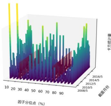
图 73 Grow_eps_dilu \chi^2 统计量分布图 (上证 50)
