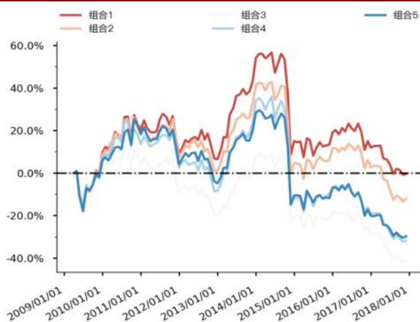
图 128 Grow_yoy_bps 分层组合走势图（上证 50）
