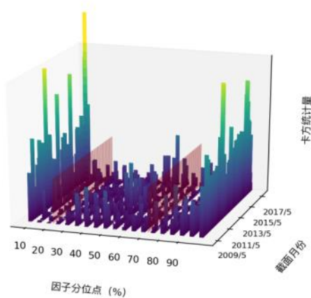
图 95 Grow_yoy_prof \chi^2 统计量分布图（沪深 300）
