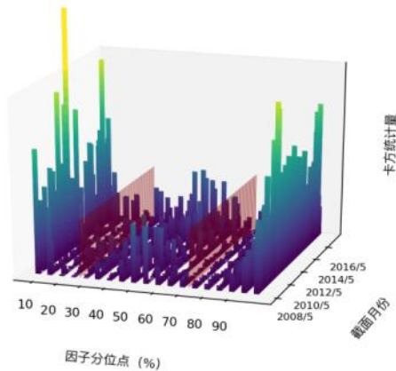
图 11 Grow_cafI_op \chi^2 统计量分布图（沪深 300）
