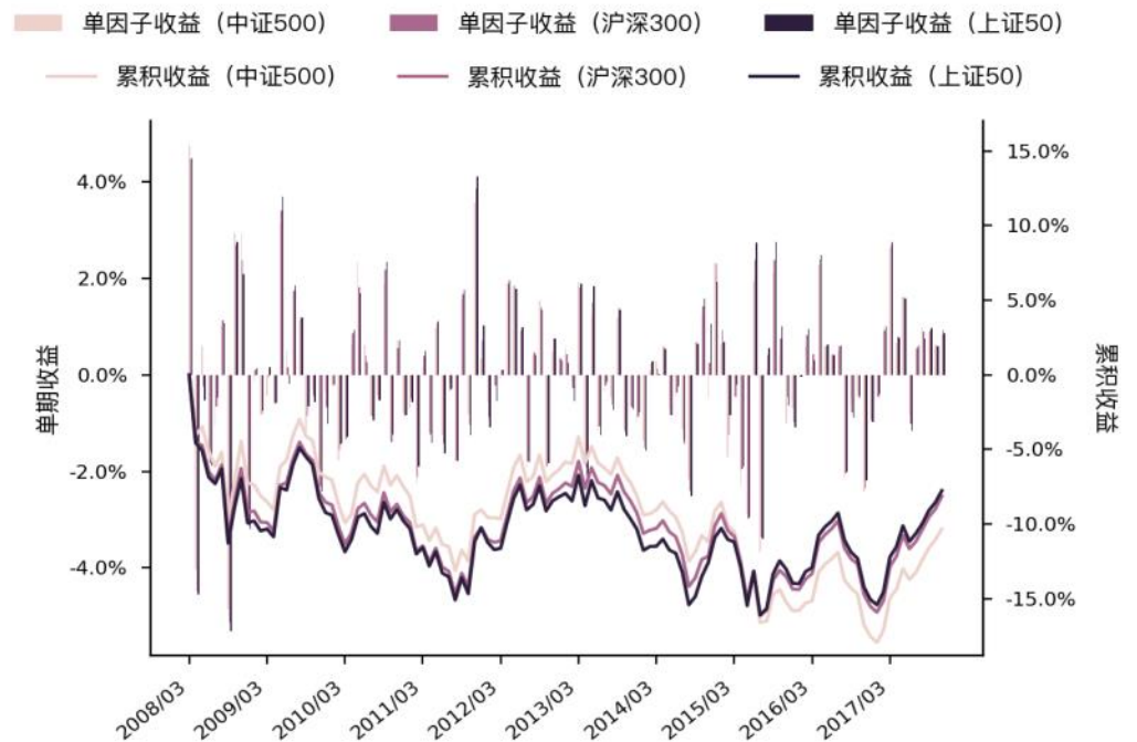
图 51 Grow_asset 单因子单期收益与累积收益图 (WLS)
