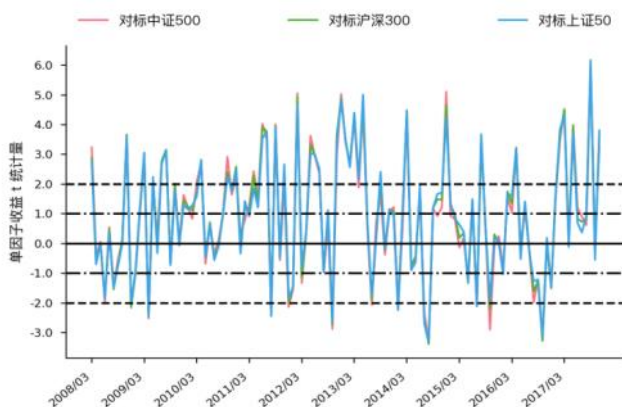
图 28 Grow_net_prof t 统计量走势图 (WLS)
