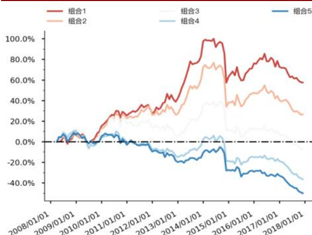
图 19 Grow_net_prof 分层组合走势图（沪深 300）
