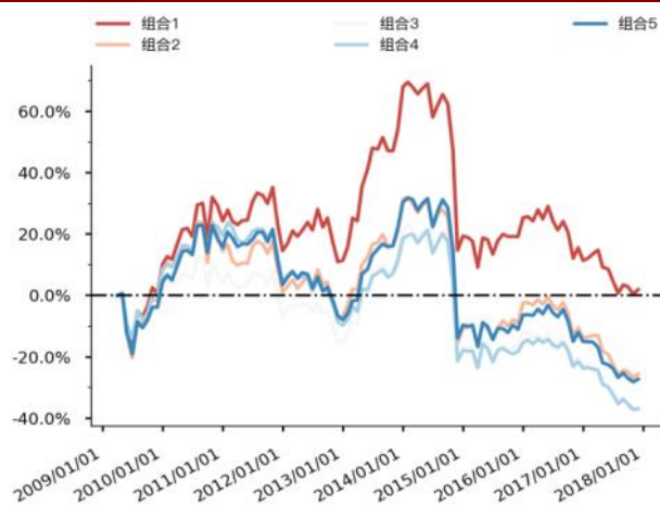
图 104 Grow_yoy_rev 分层组合走势图（上证 50）
