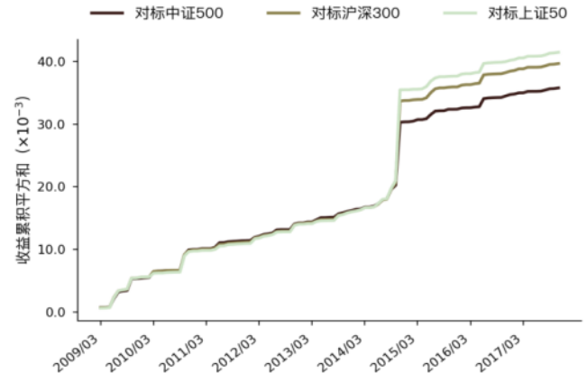
图 137 Grow_yoy_bps 因子波动量能走势图 (WLS)
