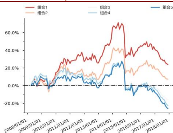
图 7 Grow_caf_l_op 分层组合走势图（沪深 300）
