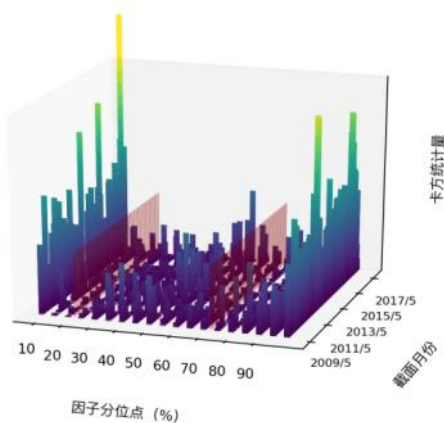
图 93 Grow_yoy_prof \chi^2 统计量分布图（中证 500）
