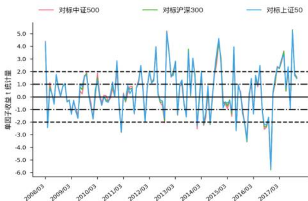
图 64 Grow_bps t 统计量走势图 (WLS)
