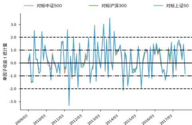
图 88 Grow_yoy_caf_l_op t 统计量走势图 (WLS)
