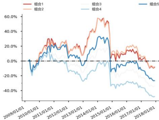
图 92 Grow_yoy_prof 分层组合走势图（上证 50）
