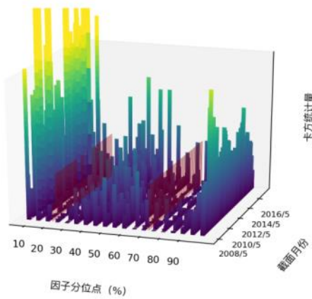
图 49 Grow_asset \chi^2 统计量分布图（上证 50）
