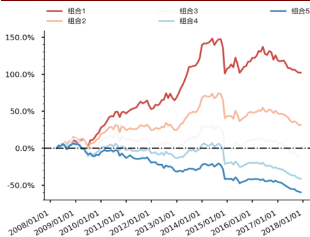
图 67 Grow_eps_dilu 分层组合走势图（沪深 300）
