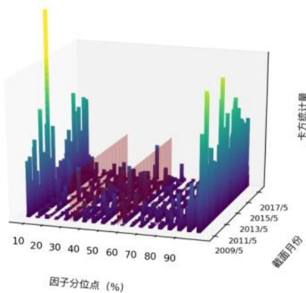
图 143 Grow_yoy_eps_dil \chi^2 统计量分布图(沪深 300) 图 144 \chi^2 统计量最小分位点走势(沪深 300)
