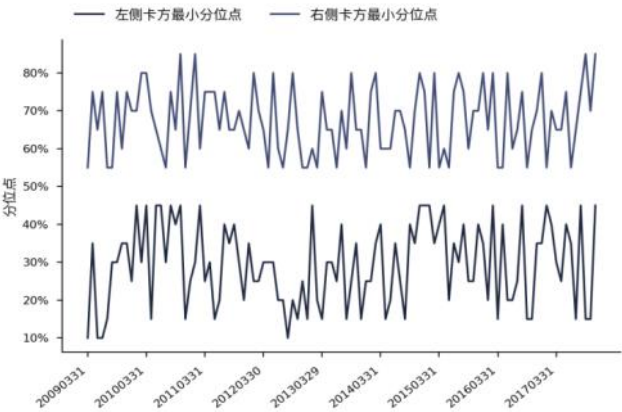
图 81 Grow_yoy_caf_l_op \chi^2 统计量分布图 (中证 500) 图 82 \chi^2 统计量最小分位点走势 (中证 500)
