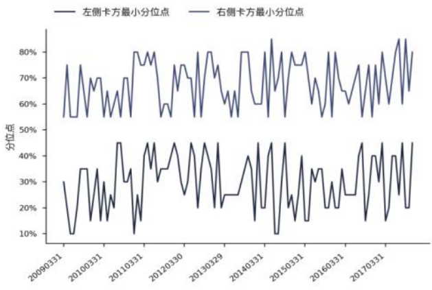
图 143 Grow_yoy_eps_dil \chi^2 统计量分布图(沪深 300) 图 144 \chi^2 统计量最小分位点走势(沪深 300)
