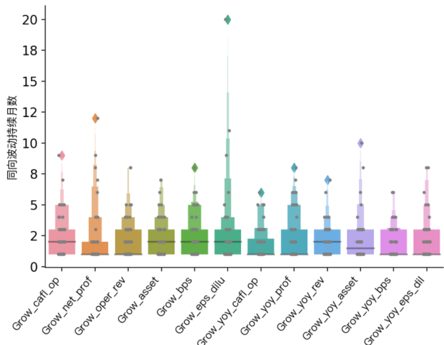
图 150 成长类因子同向波动持续月份数分布 (中证 500)
