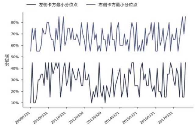
图 83 Grow_yoy_caf1_op \chi^2 统计量分布图 (沪深 300) 图 84 \chi^2 统计量最小分位点走势 (沪深 300)
