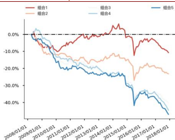
图 6 Grow_caf_l_op 分层组合走势图（中证 500）
