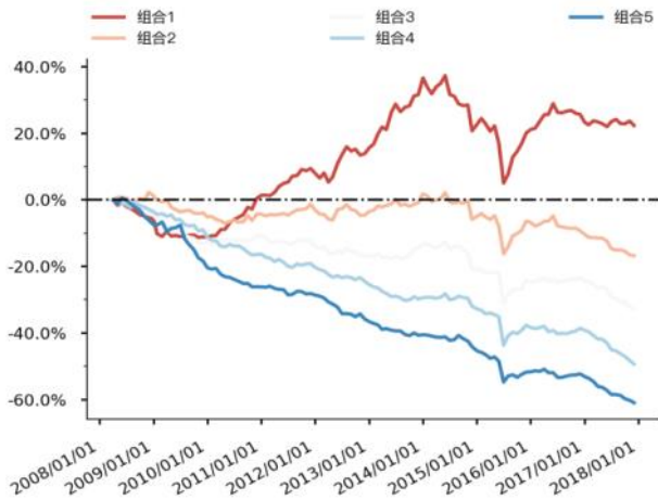
图 30 Grow_oper_rev 分层组合走势图（中证 500）
