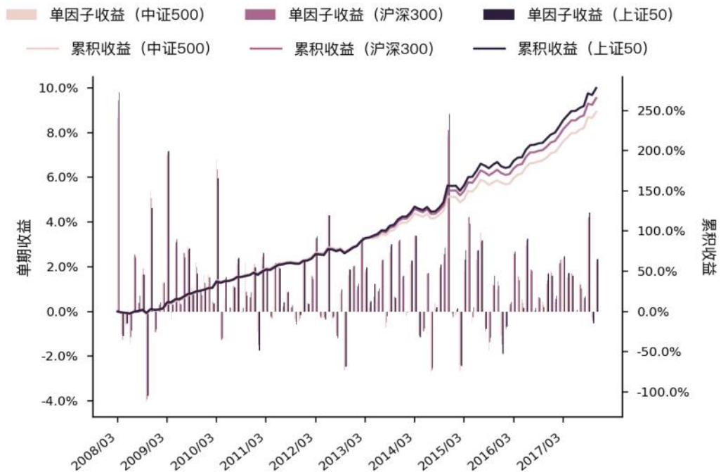
图 75 Grow_eps_dilu 单因子单期收益与累积收益图 (WLS)
