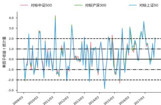
图 124 Grow_yoy_asset t 统计量走势图 (WLS)
