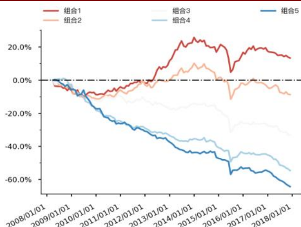
图 18 Grow_net_prof 分层组合走势图（中证 500）
