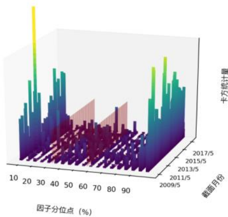
图 141 Grow_yoy_eps_dil \chi^2 统计量分布图(中证 500)
