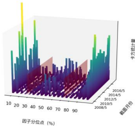
图 13 Grow_cafI_op \chi^2 统计量分布图（上证 50）
