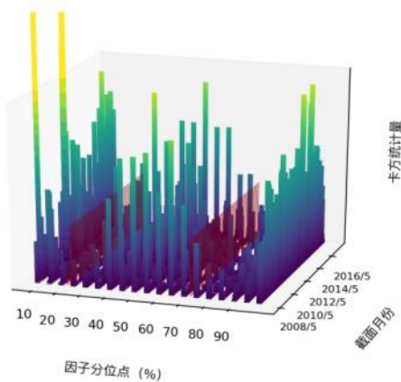
图 71 Grow_eps_dilu \chi^2 统计量分布图 (沪深 300)
