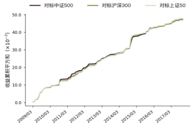
图 101 Grow_yoy_prof 因子波动量能走势图 (WLS)
