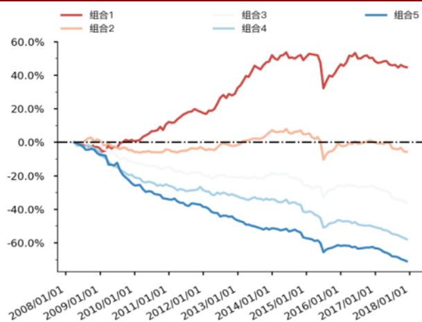
图 66 Grow_eps_dilu 分层组合走势图（中证 500）
