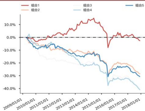
图 102 Grow_yoy_rev 分层组合走势图（中证 500）
