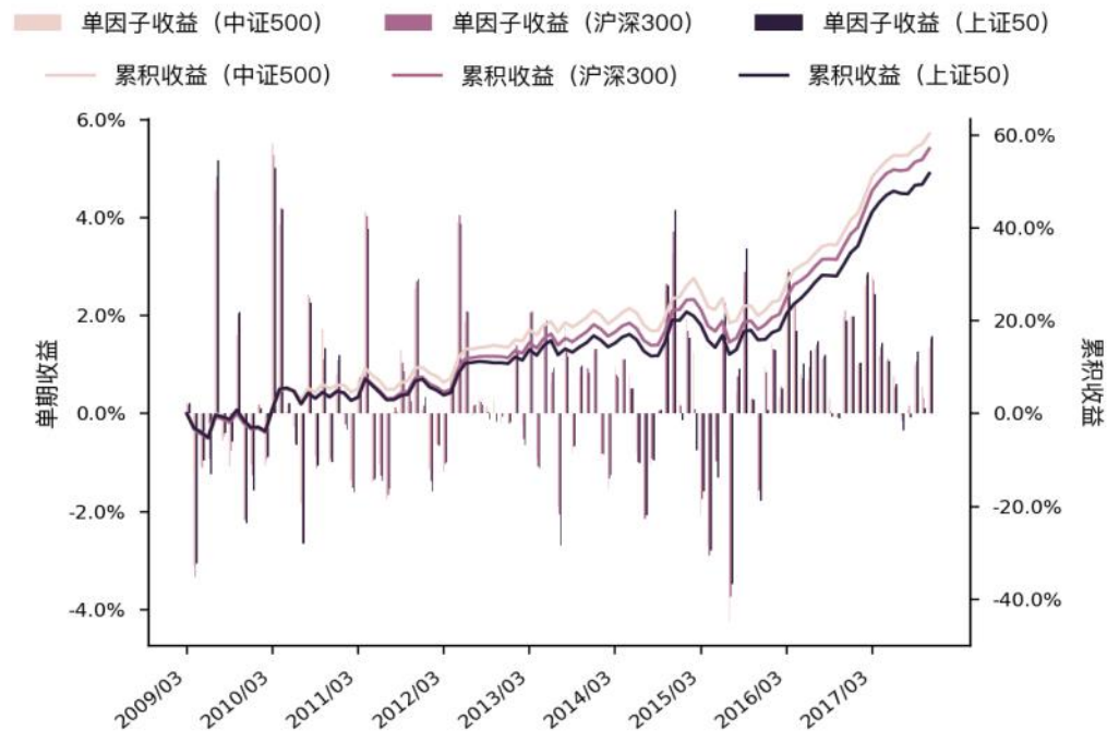
图 123 Grow_yoy_asset 单因子单期收益与累积收益图 (WLS)
