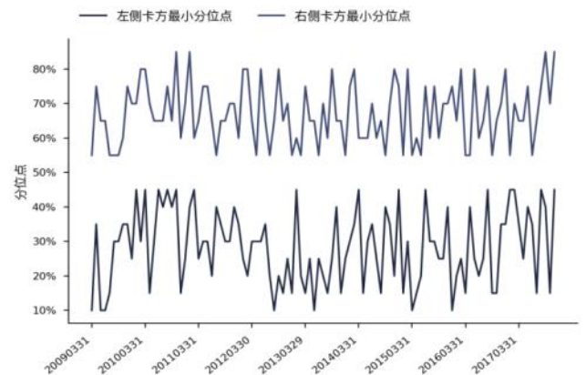
图 85 Grow_yoy_caf1_op \chi^2 统计量分布图 (上证 50) 图 86 \chi^2 统计量最小分位点走势 (上证 50)
