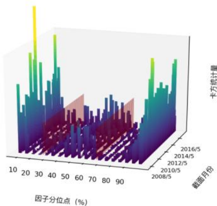
图 9 Grow_cafI_op \chi^2 统计量分布图（中证 500）
