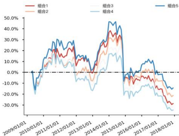
图 140 Grow_yoy_eps_dil 分层组合走势图（上证 50）
