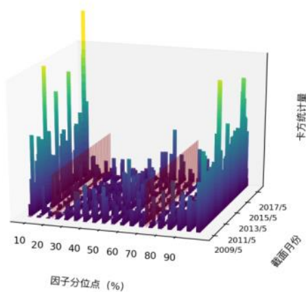
图 97 Grow_yoy_prof \chi^2 统计量分布图（上证 50）
