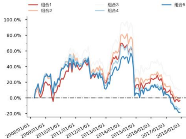
图 44 Grow_asset 分层组合走势图（上证 50）
