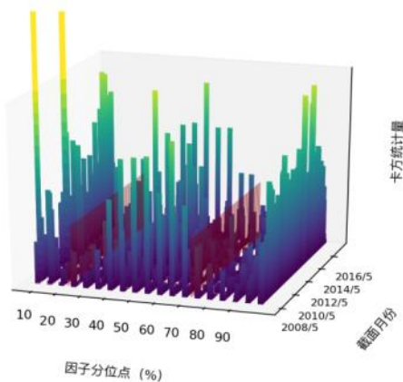
图 69 Grow_eps_dilu \chi^2 统计量分布图（中证 500）
