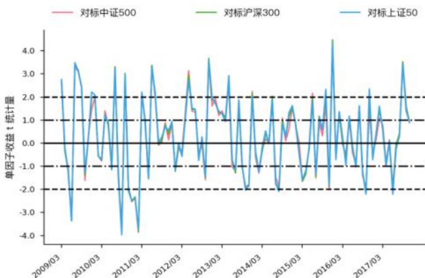
图 112 Grow_yoy_rev t 统计量走势图 (WLS)
