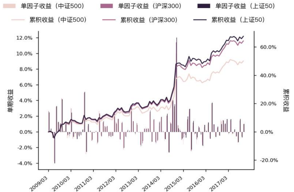
图 135 Grow_yoy_bps 单因子单期收益与累积收益图 (WLS)
