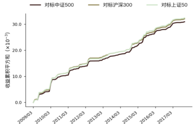
图 125 Grow_yoy_asset 因子波动量能走势图 (WLS)
