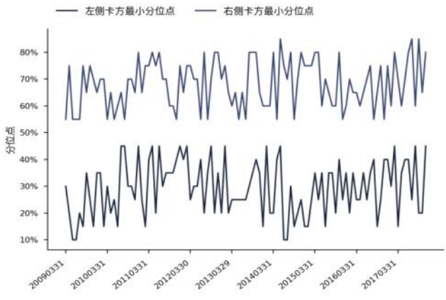
图 145 Grow_yoy_eps_dil \chi^2 统计量分布图(上证 50) 图 146 \chi^2 统计量最小分位点走势(上证 50)
