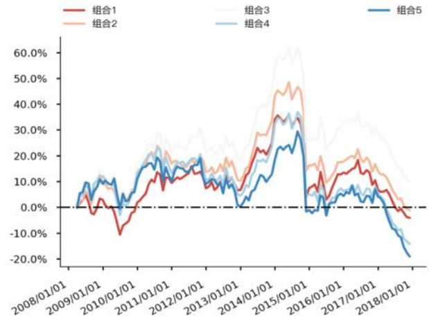
图 43 Grow_asset 分层组合走势图（沪深 300）
