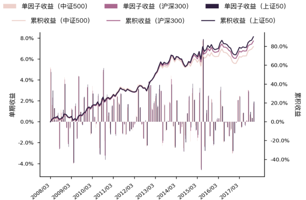
图 39 Grow_oper_rev 单因子单期收益与累积收益图 (WLS)
