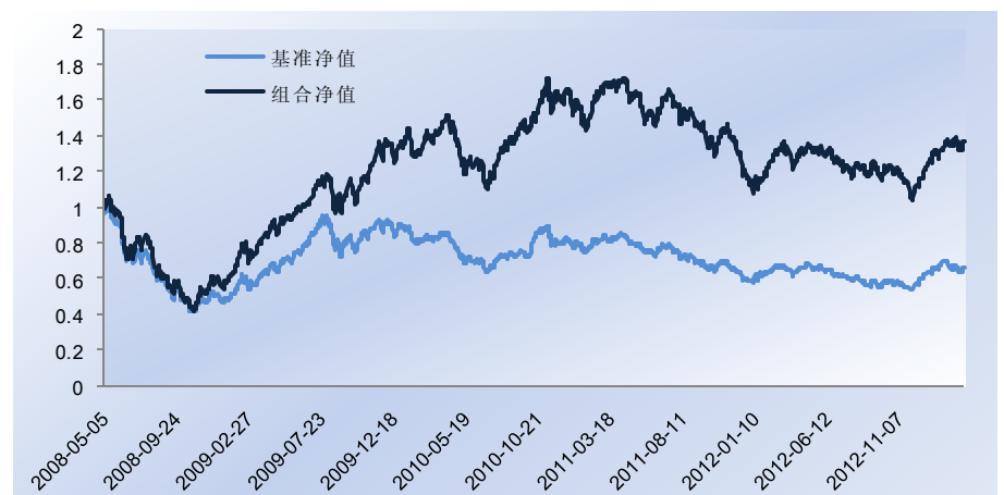
图 5：最优拟合组合收益与沪深 300 收益对比（20080430 - 20130322）
