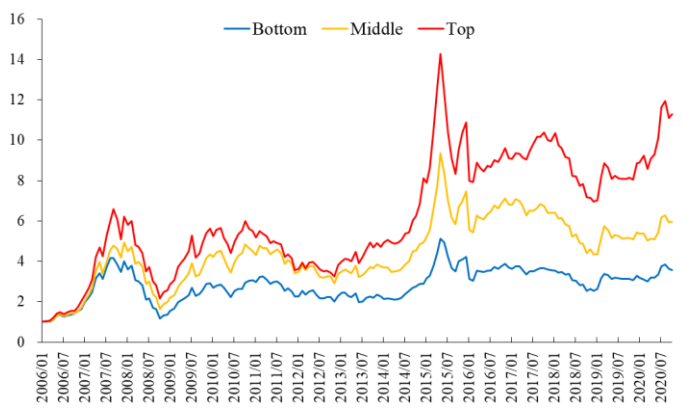
图6：日内因子 M0 分组表现（200601-202010）
