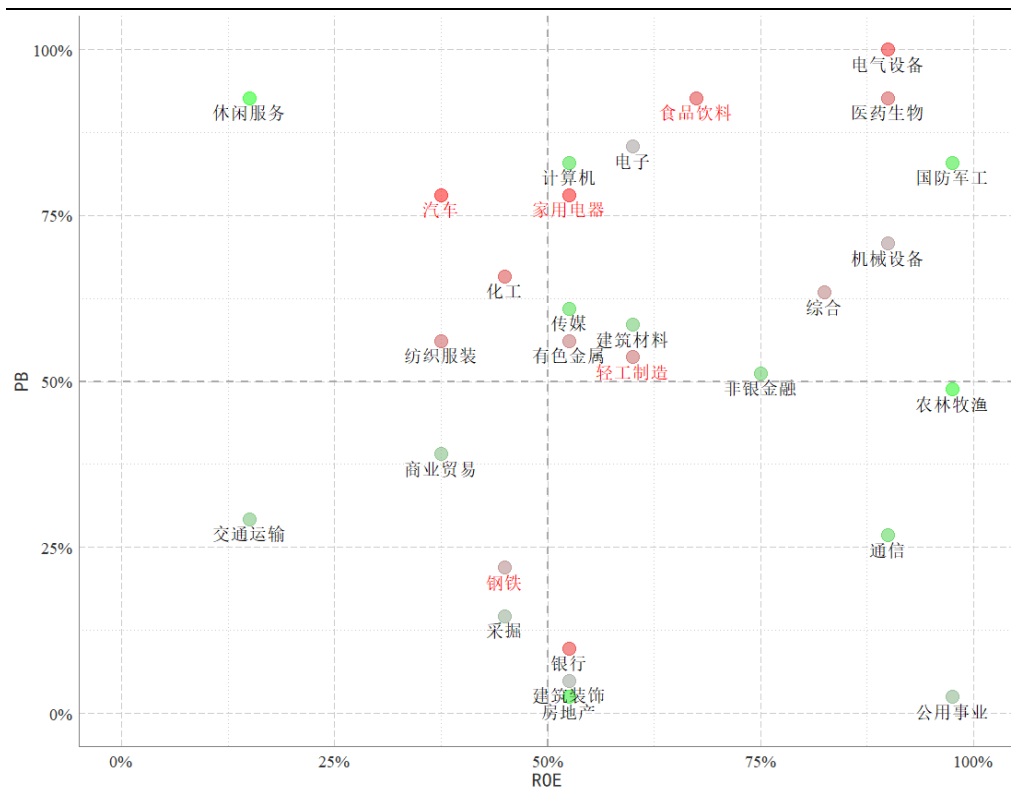
图18: 行业PB-ROE历史分位点(20201031)
