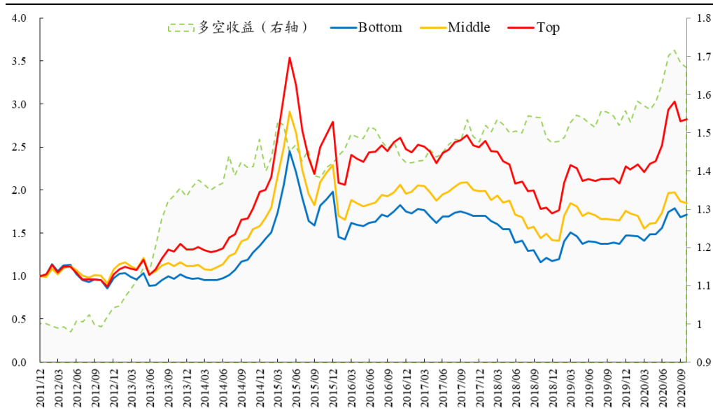
图10：行业龙头股模型三分组表现（201201~202010）
