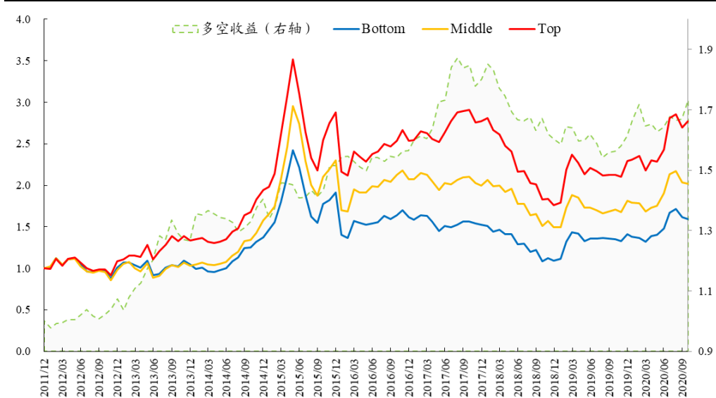
图8：行业黄金律模型三分组表现（201201~202010）
