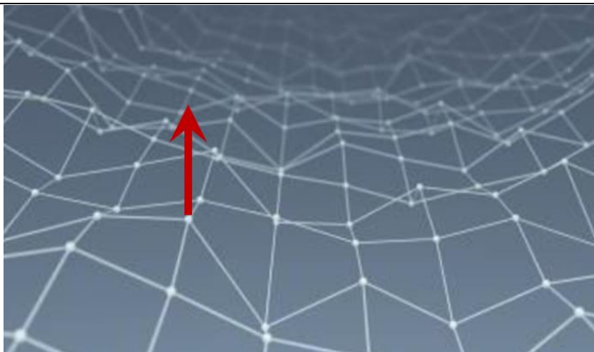
图9：龙头股与普通股动量传导示意图
