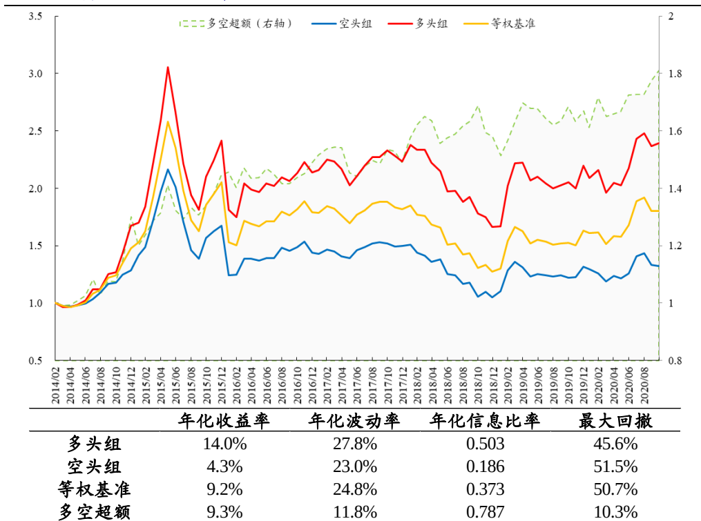
图20: 强势板块优选历史表现 (201402-202010)
