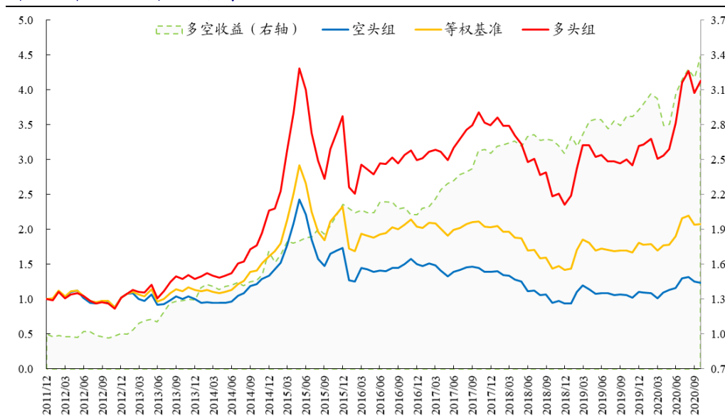
图 16: 开源金工行业配置表现 (2012Q1~2020Q9)
