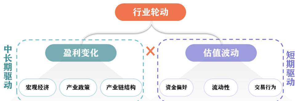
图3: 行业轮动现象
