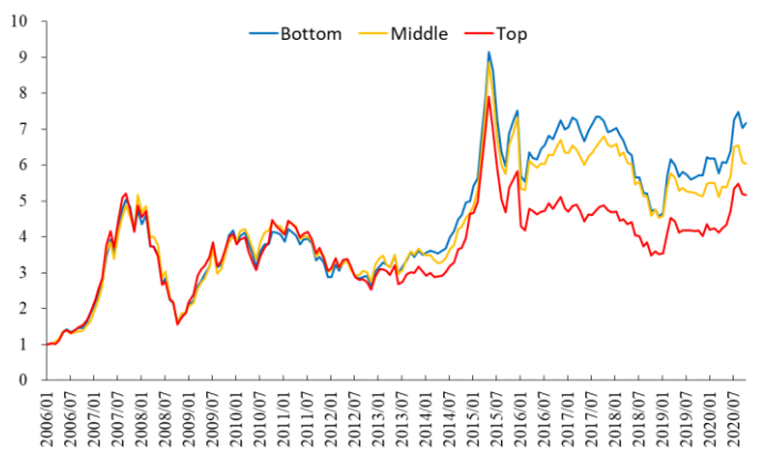
图7：隔夜因子 M1 分组表现（200601-202010）
