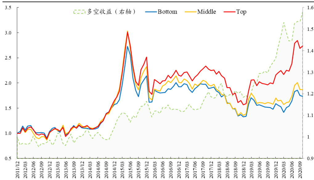
图 11：行业景气度模型三分组表现（201201~202010）
