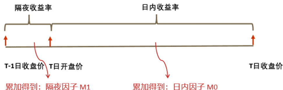
图5：隔夜因子与日内因子拆分示意图
