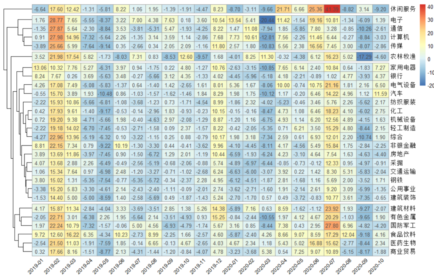
图2：28 个行业月度收益聚类（201901-202010）
