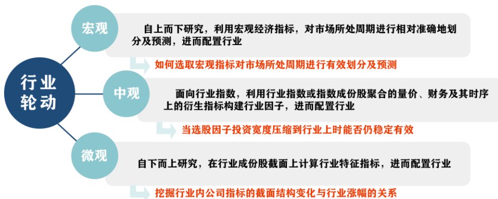
图4: 行业轮动的研究视角
