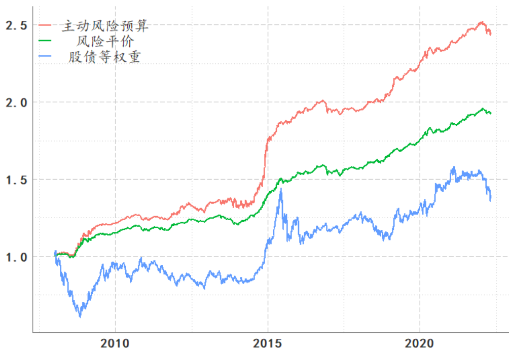
图5：主动风险预算组合净值走势（年化收益6.63%，收益波动比1.67）
