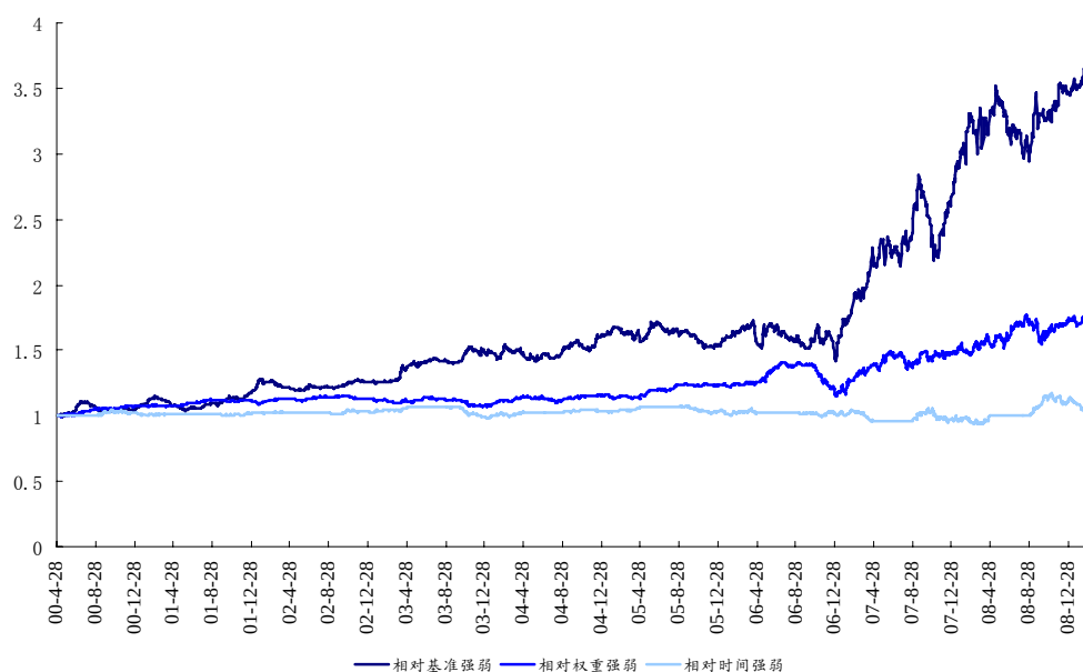
图 4 RVmoye 指数与其他指数相对强弱的比较
