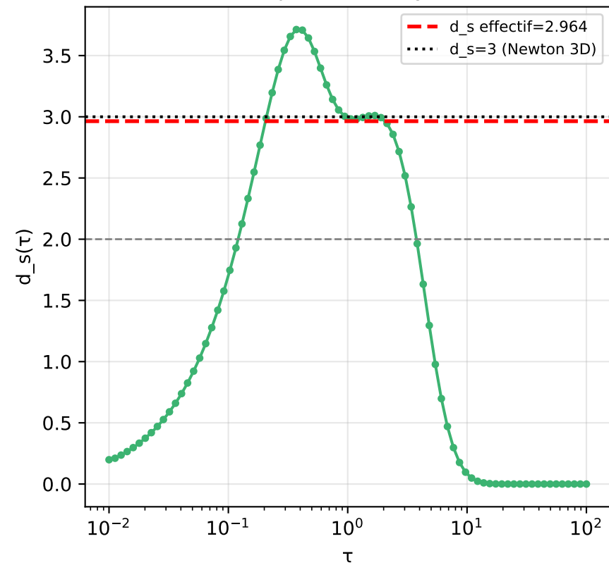
Dimension spectrale (noyau chaleur)
