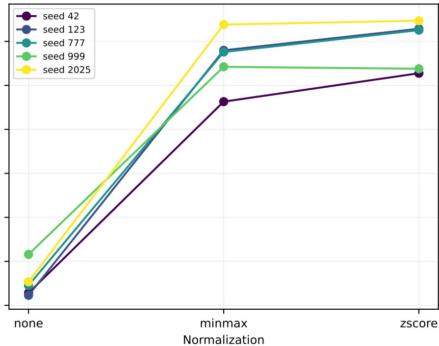
Static GCN
