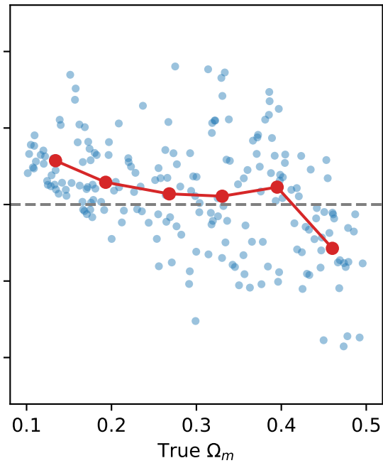
GCN-GRU Seed 123
