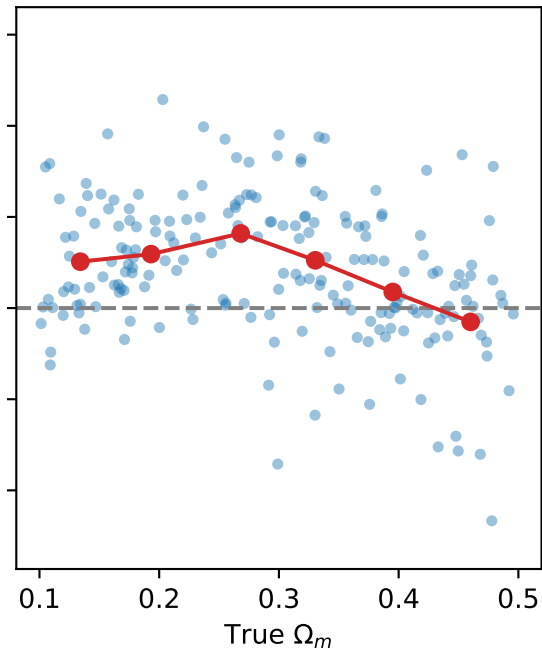
EvolveGCN-O Seed 123
