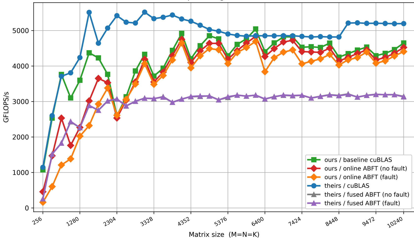
GFLOPS — Square, big ( M=N=K , 256-10240)
