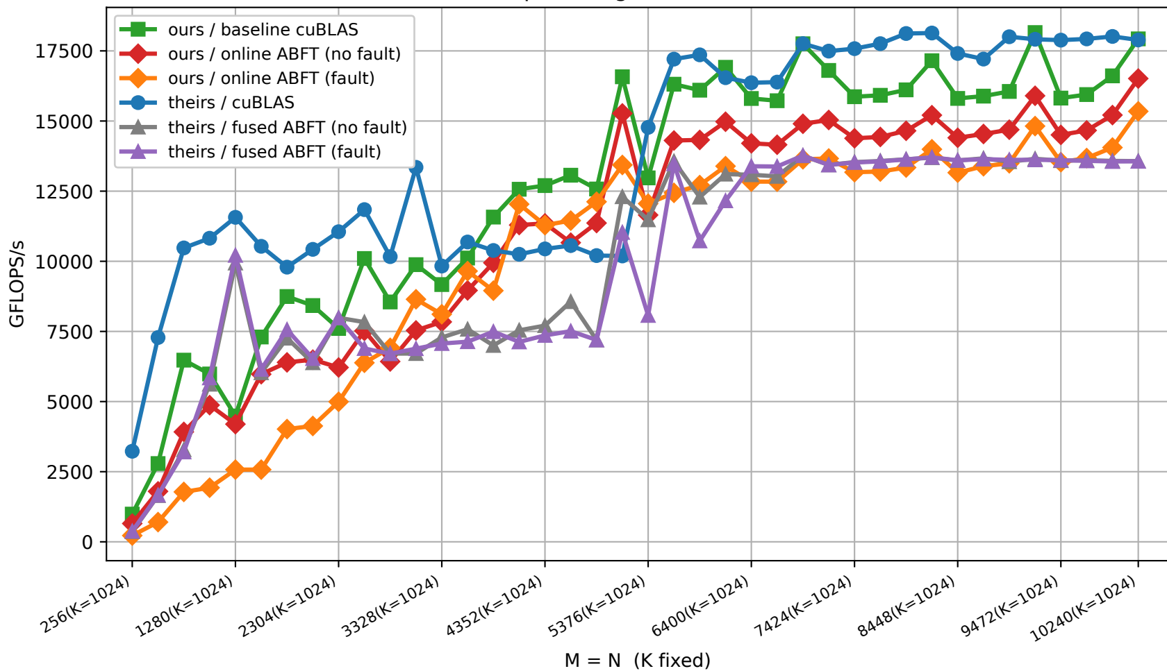
GFLOPS — Non-square, big ( M=N , K=1024 , 256-10240)
