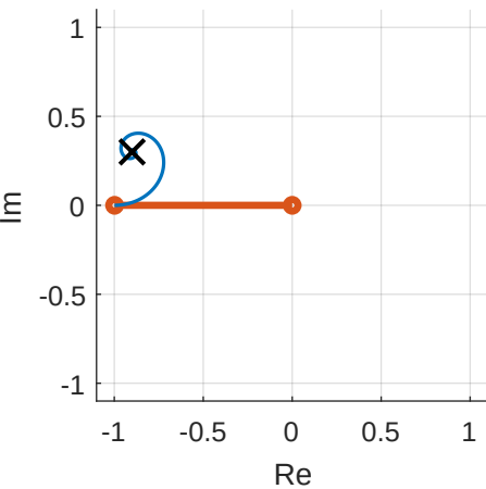
(d) \Delta f_{\text{detune}} = +1.5\Delta\nu_{\text{FWHM}}
