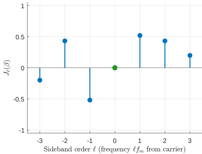
Carrier null: \beta = 2.405 , J_0J_1 = -0.000
