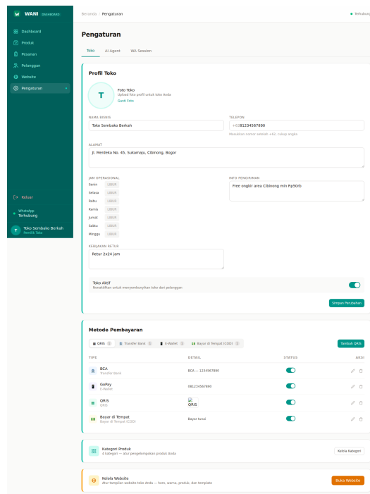
Gambar 12: Pengaturan Toko
