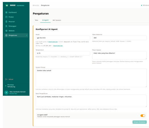
Gambar 13: Pengaturan AI
