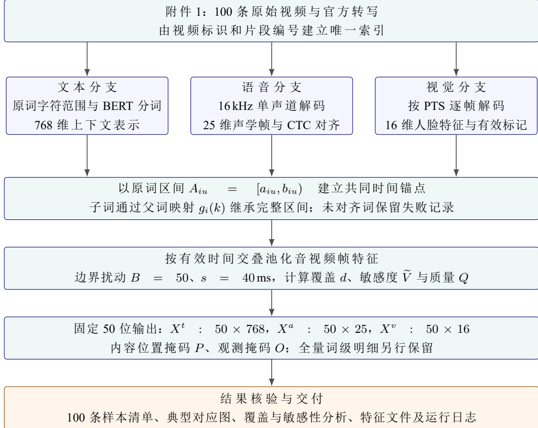
图 2 三模态特征提取与时间锚点对齐流程。声学特征与强制对齐共用音频信号；视觉帧采用自身解码时间戳。
