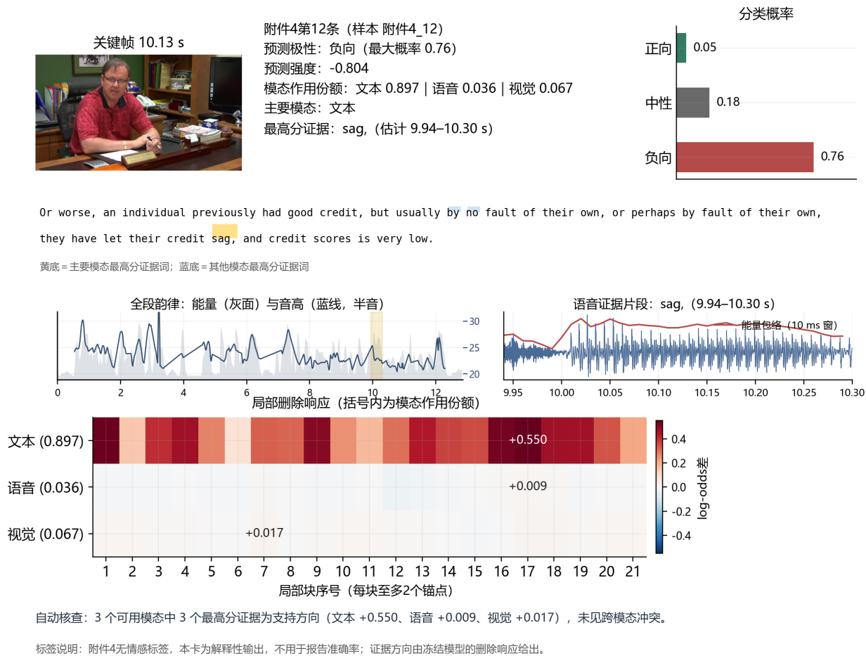
图 21 附件 4 第 12 条 (转折样本) 解释卡
