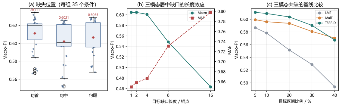
图 12 缺失位置、缺口长度与基线比较
