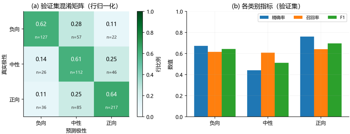
图 17 验证集混淆矩阵与分类指标
