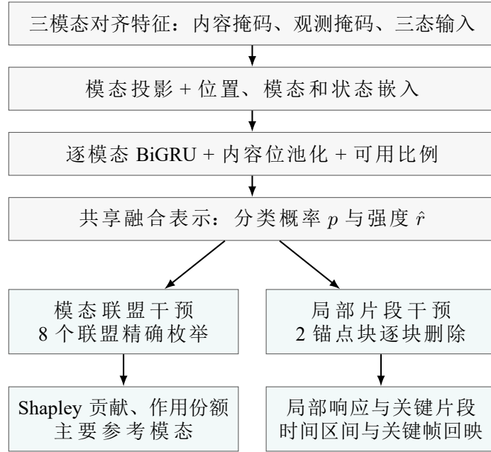
图 16 问题三 ICF-Shapley 预测器与解释层结构
