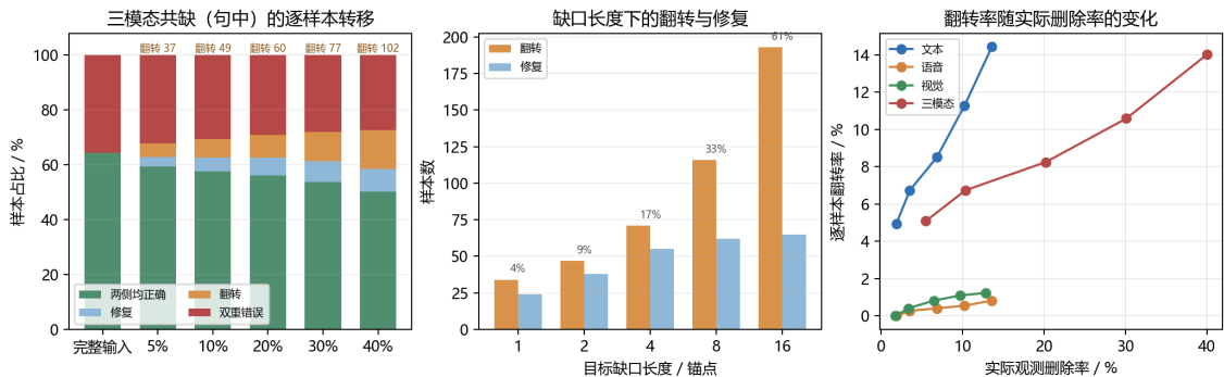
图 13 受控缺口下的逐样本错误转移
